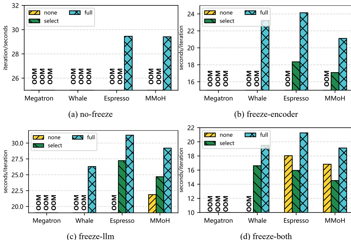
图 4.4 不同冻结策略下各框架迭代时间对比（自左至右、自上至下依次为 no-freeze、freeze-encoder、freeze-llm、freeze-both）。
