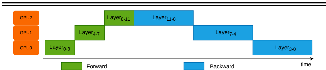
图 2.4 流水线并行示意
