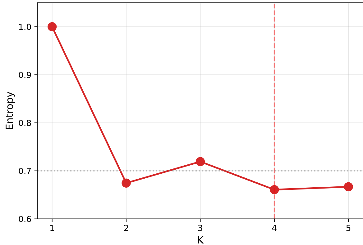
B. Entropy ( \geq 0.7 = good)
