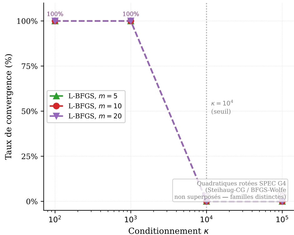
Figure §5 — L-BFGS vs Steihaug-CG / BFGS-Wolfe sur problèmes mal conditionnés (Cat. A)
