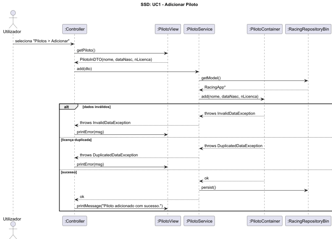
Figura 3: SSD UC1 - Adicionar Piloto.
