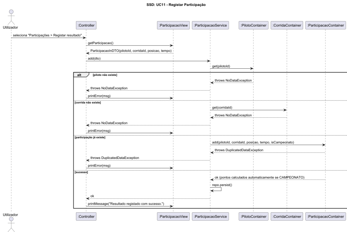
Figura 5: SSD UC11 - Registrar Participação.
