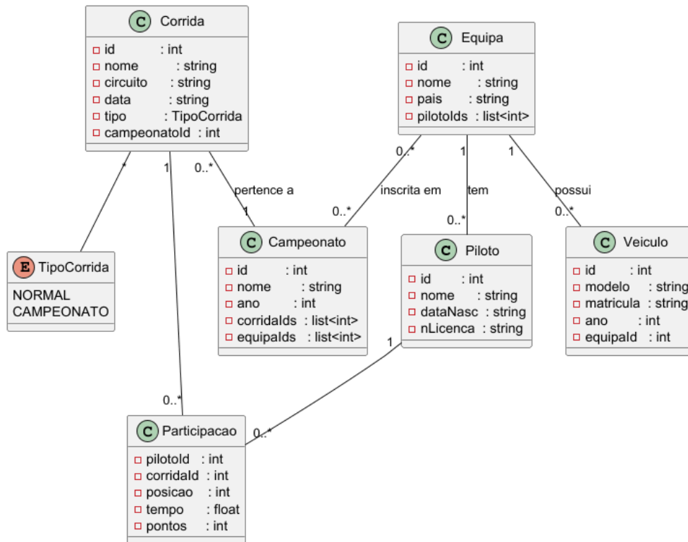
Figura 2: Modelo de domínio do sistema.
