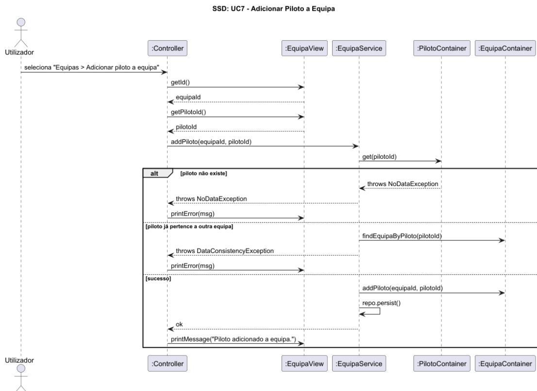
Figura 4: SSD UC7 - Adicionar Piloto a Equipa.
