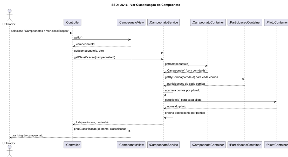
Figura 6: SSD UC16 - Ver Classificação do Campeonato.
