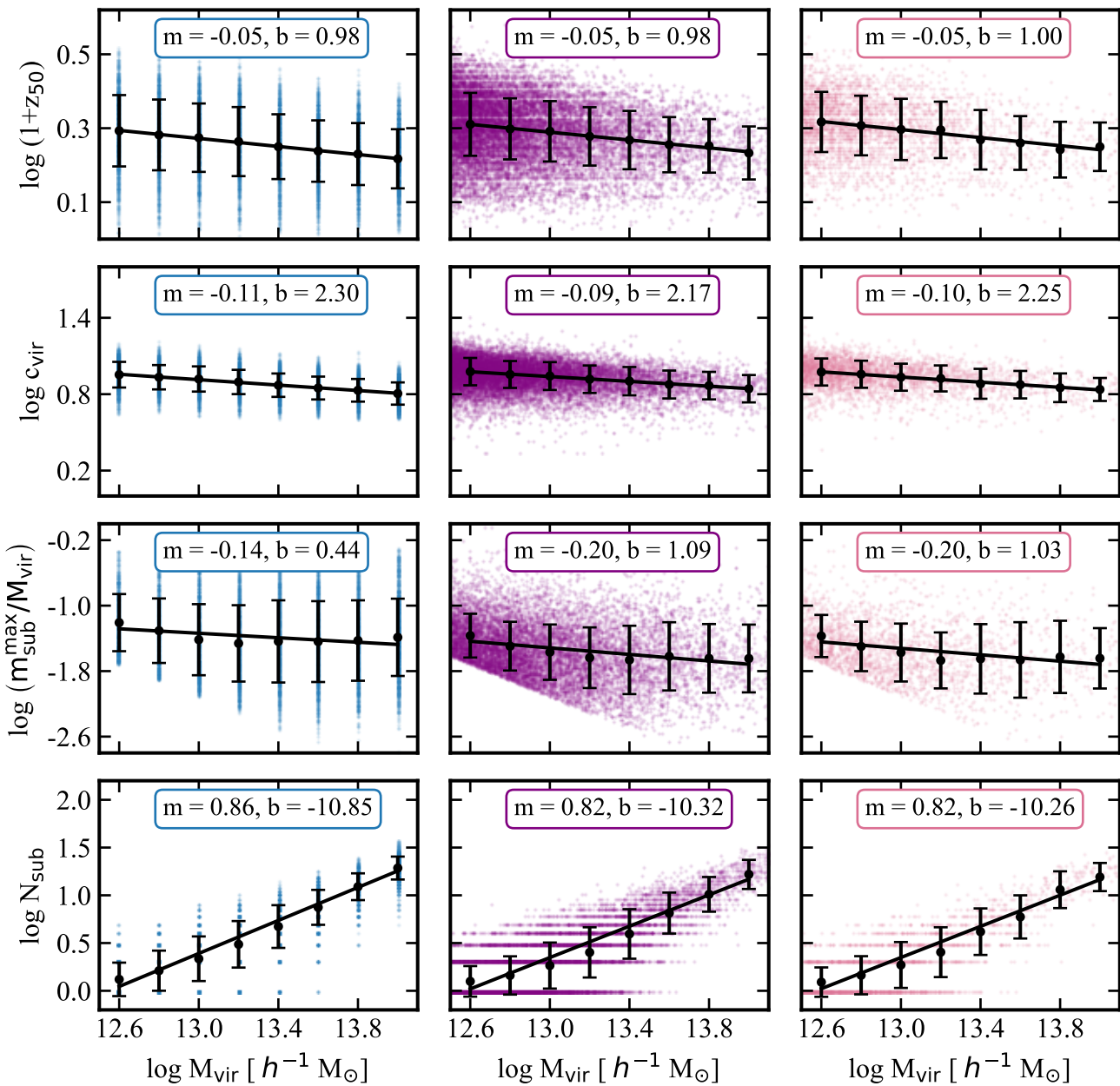
SatGen
