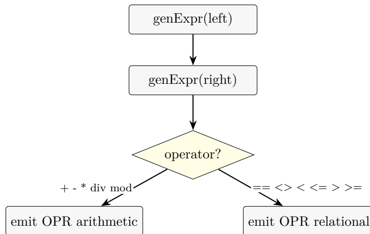
Figure 2: Skema translasi ekspresi biner pada code generator.
