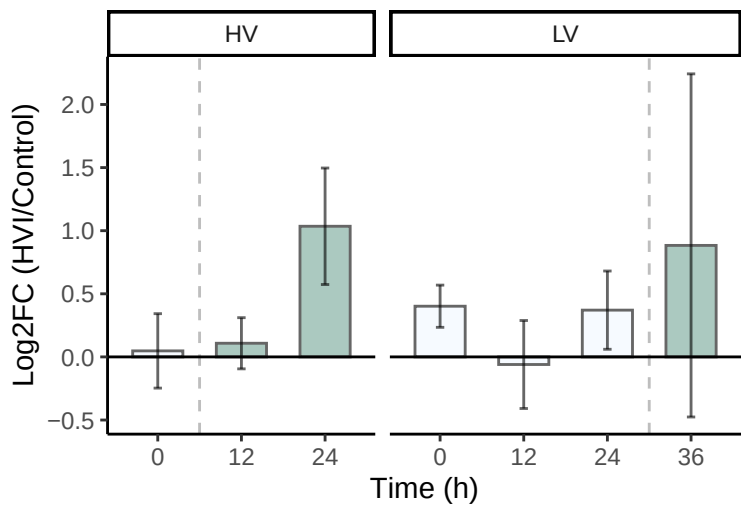
S-Adenosylmethionine
