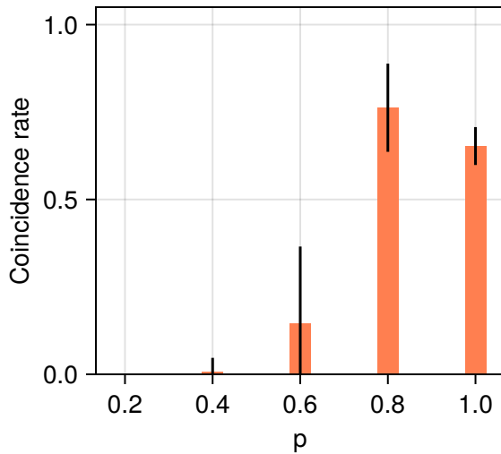
SQA
