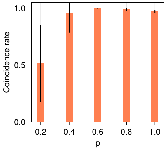
SA
