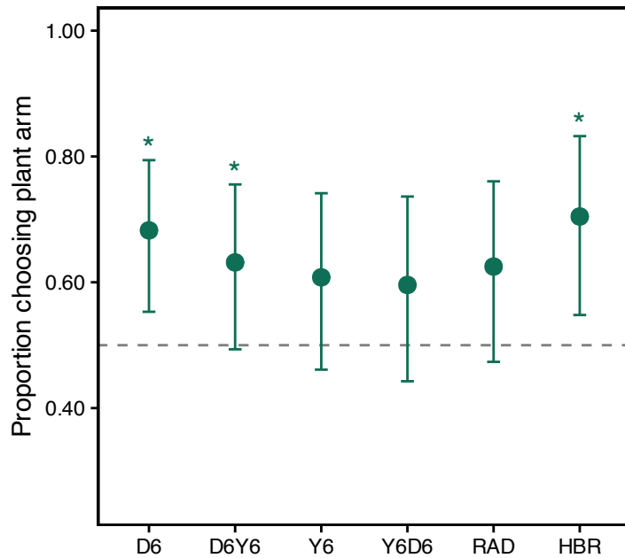
M. janthiniformis
