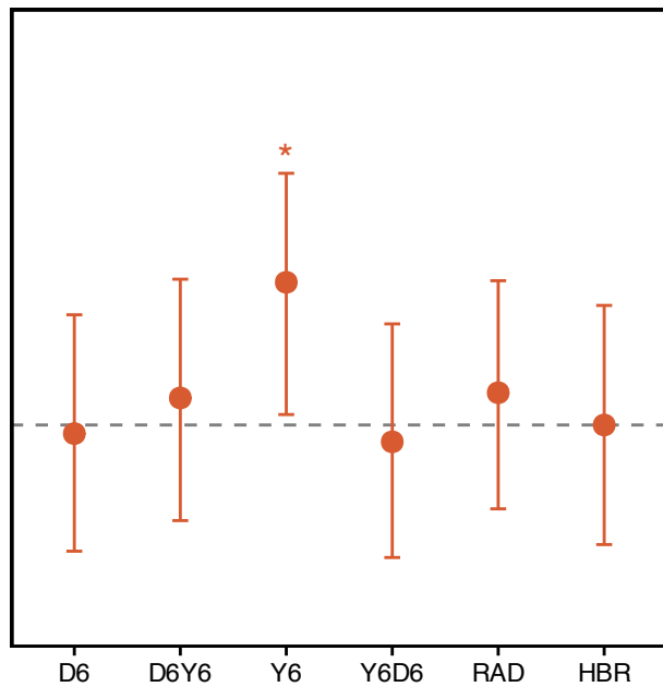
M. janthinus
