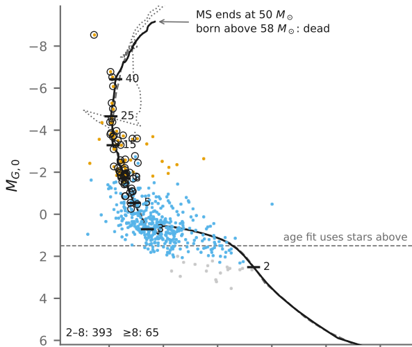
Cyg OB2-A PARSEC 4.01 Myr · MIST 4.05 Myr
