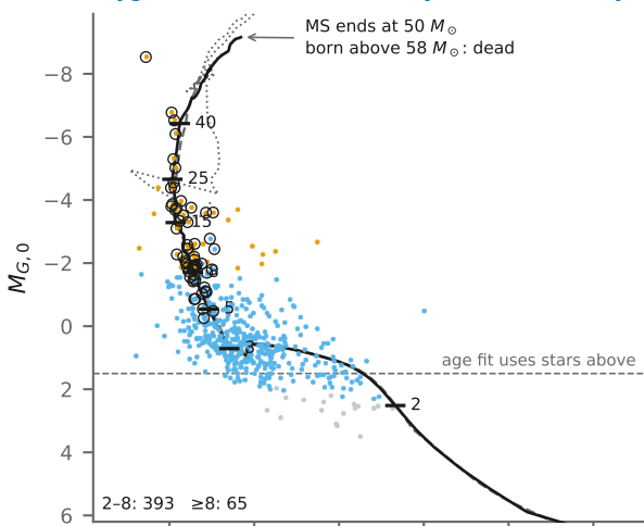
Cyg OB2-A PARSEC 4.01 Myr · MIST 4.05 Myr
