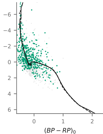
Cyg OB2-C 2.52 Myr
