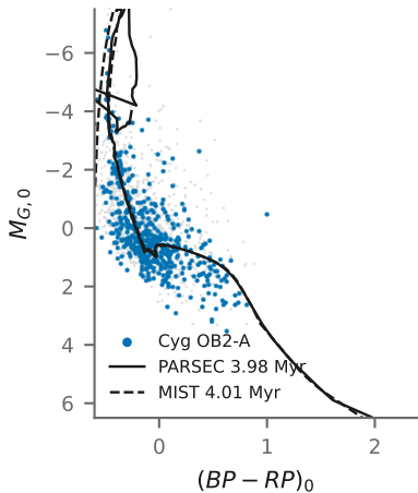
Cyg OB2-A 4.01 Myr
