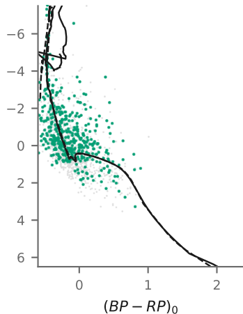
Cyg OB2-C 3.38 Myr
