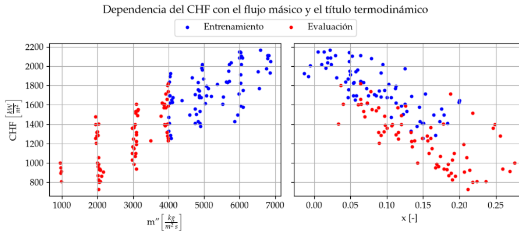
FIGURA 4.11. División de los datos de CHF de la Universidad de Columbia en entrenamiento y evaluación, según flujo másico. Los ejes de flujo másico y título termodinámico corresponden a los valores promedios de la sección de ensayo a la salida.
