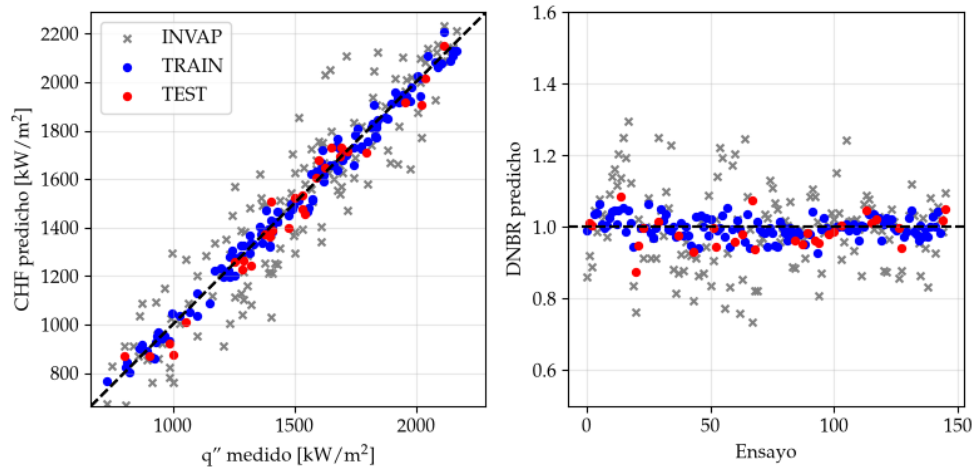
FIGURA 4.28. CHF predicho contra real y DNB por ensayo para modelo final MFP INN.
