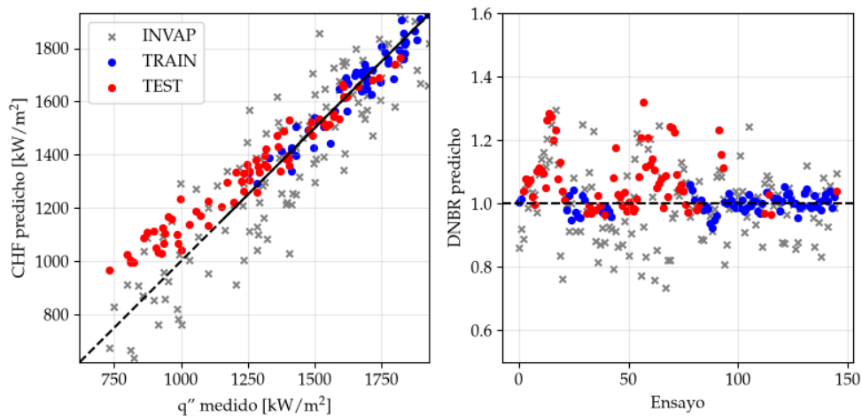
FIGURA 4.24. CHF predicho contra real y DNBR por ensayo, para MFDDNN con variables de entrada expandidas.
