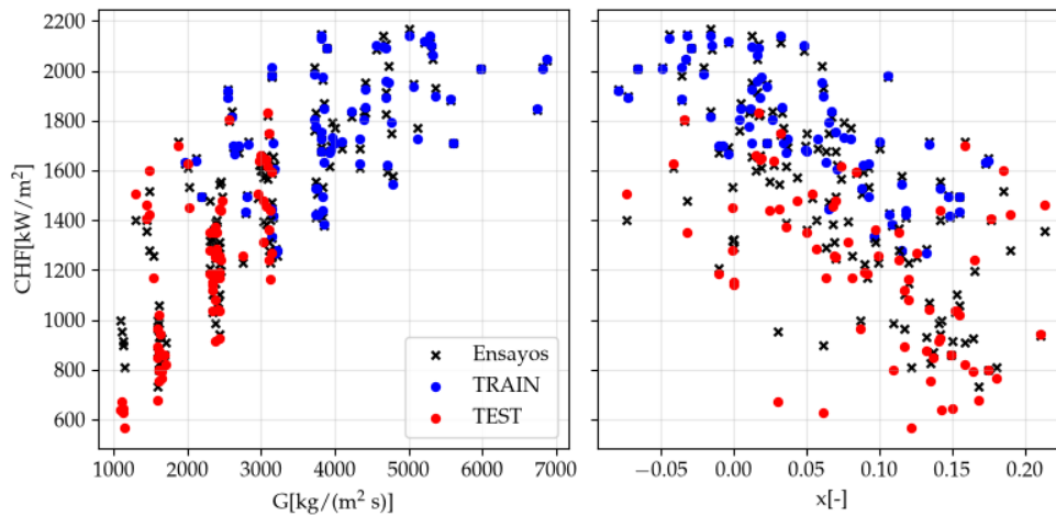
FIGURA 4.23. Relación de CHF con el flujo másico y el título termodinámico para variante D de MFPIINN, con variables de entrada expandidas.
