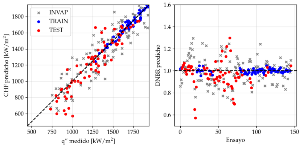
FIGURA 4.16. CHF predicho contra medido y DNBR por ensayo para variante A de \text{MFP INN} .
