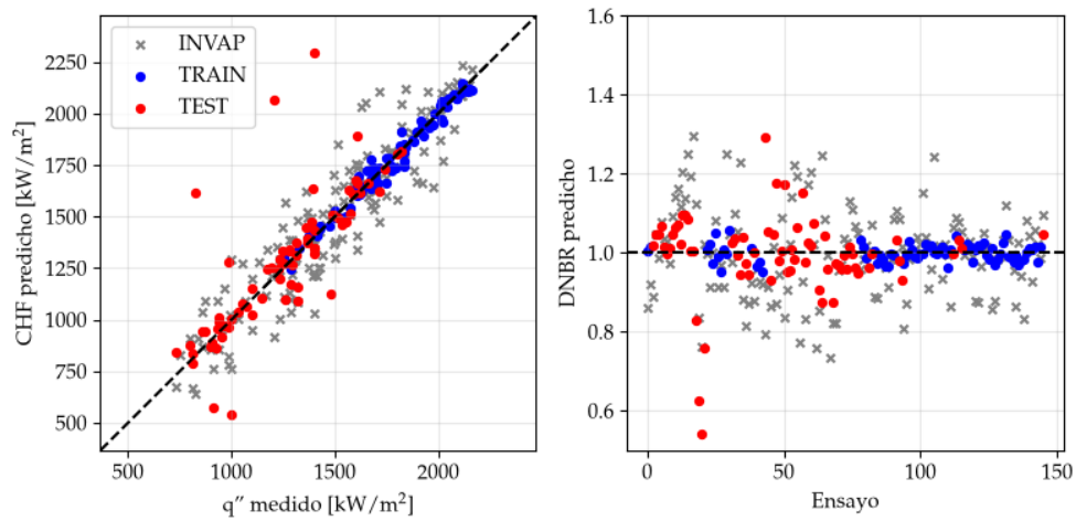
FIGURA 4.18. CHF predicho contra medido y DNBR por ensayo para variante D de MFP INN.
