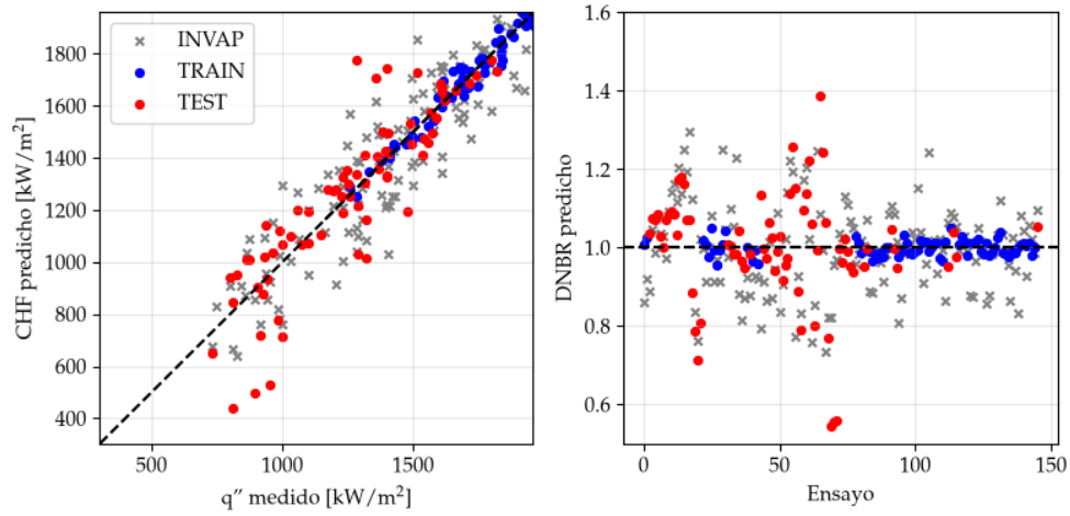
FIGURA 4.17. CHF predicho contra medido y DNBR por ensayo para variante B de MFP INN.
