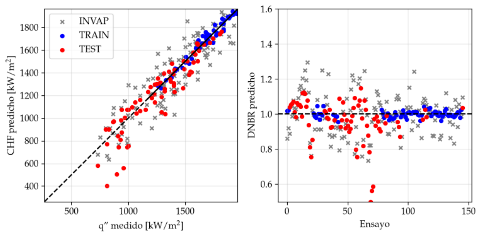
FIGURA 4.19. CHF predicho contra medido y DNBR por ensayo para variante E de MFP INN.
