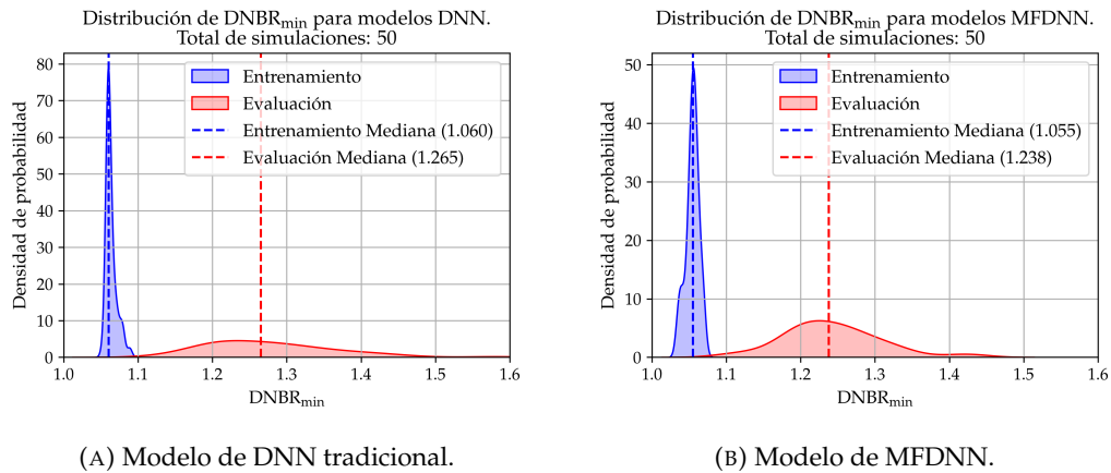
FIGURA 4.14. Distribución de probabilidad de \text{DNBR}_{\min} para N = 50 modelos entrenados de cada tipo.
