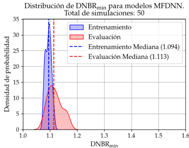
FIGURA 4.26. Distribución de densidad de probabilidad de DNBR_{min} para 50 modelos MFDNN entrenados.
