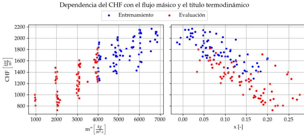
FIGURA 4.12. División de los datos de CHF de la Universidad de Columbia en entrenamiento y evaluación, según flujo másico. Los ejes de flujo másico y título termodinámico corresponden a los valores promedios de la sección de ensayo a la salida.
