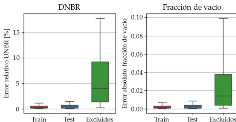
FIGURA 4.4. Distribución del error para cada objetivo, por conjunto de datos.
