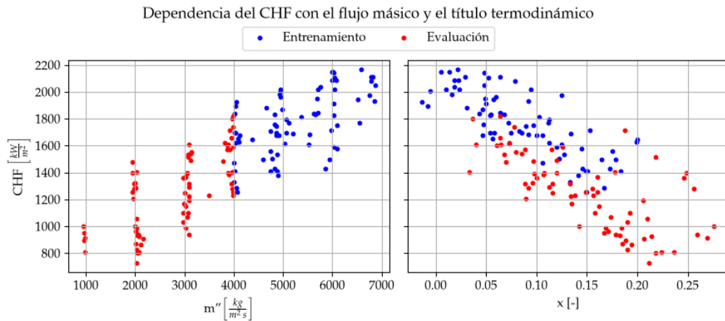
FIGURA 4.8. División de los datos de CHF de la Universidad de Columbia en entrenamiento y evaluación, según flujo másico.
