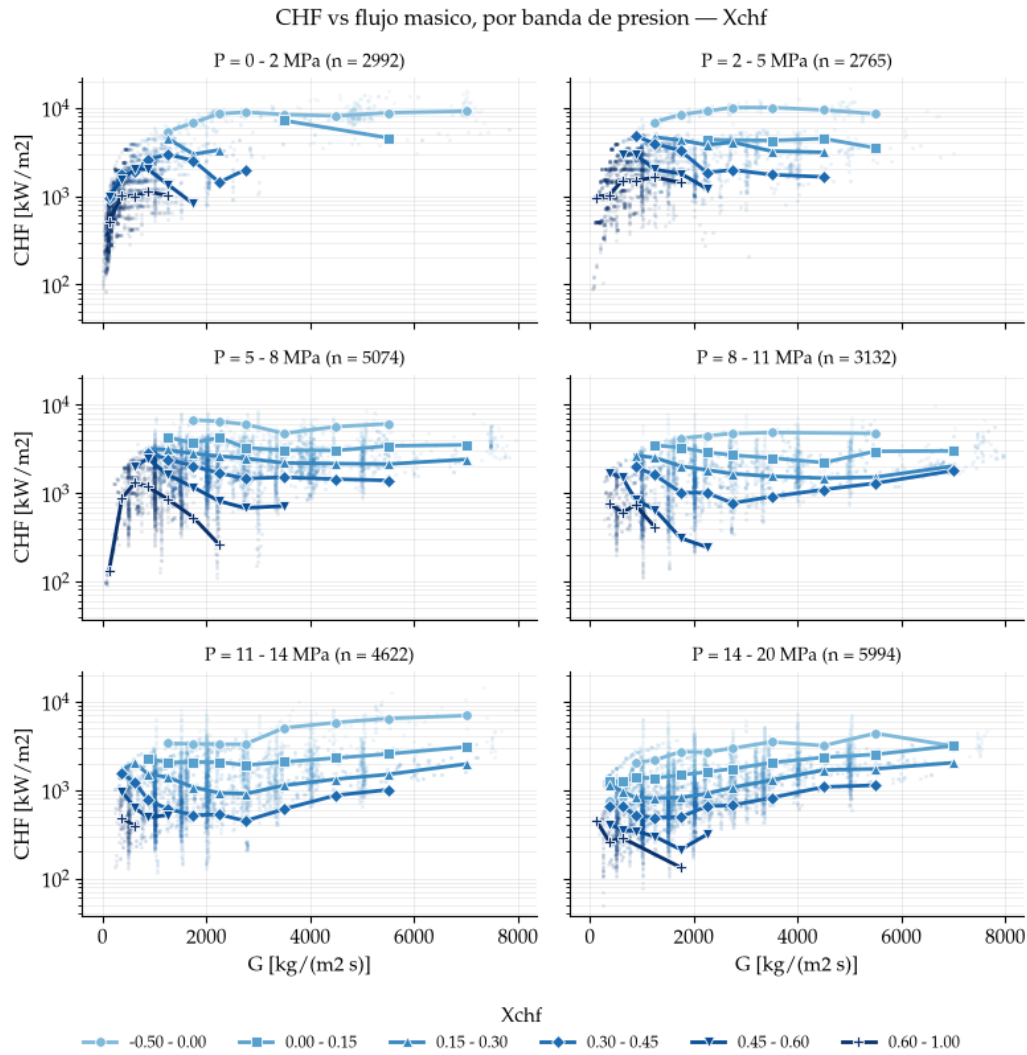
FIGURA 3.7. Tendencia del CHF con el flujo másico, para los datos de los ensayos en un tubo recopilados por Groeneveld [27, 9].
