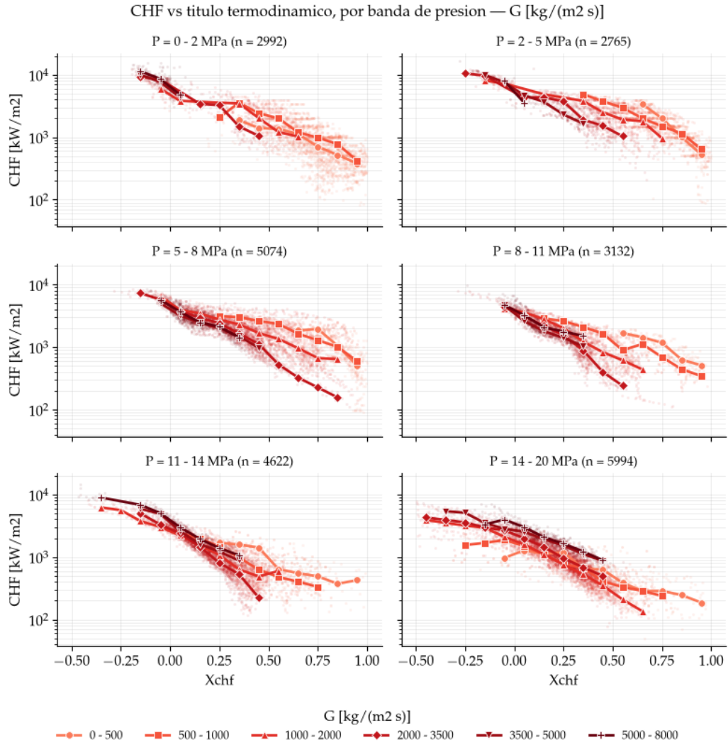
FIGURA 3.8. Tendencia del CHF con el título termodinámico, para los datos de los ensayos en un tubo recopilados por Groeneveld [27, 9].
