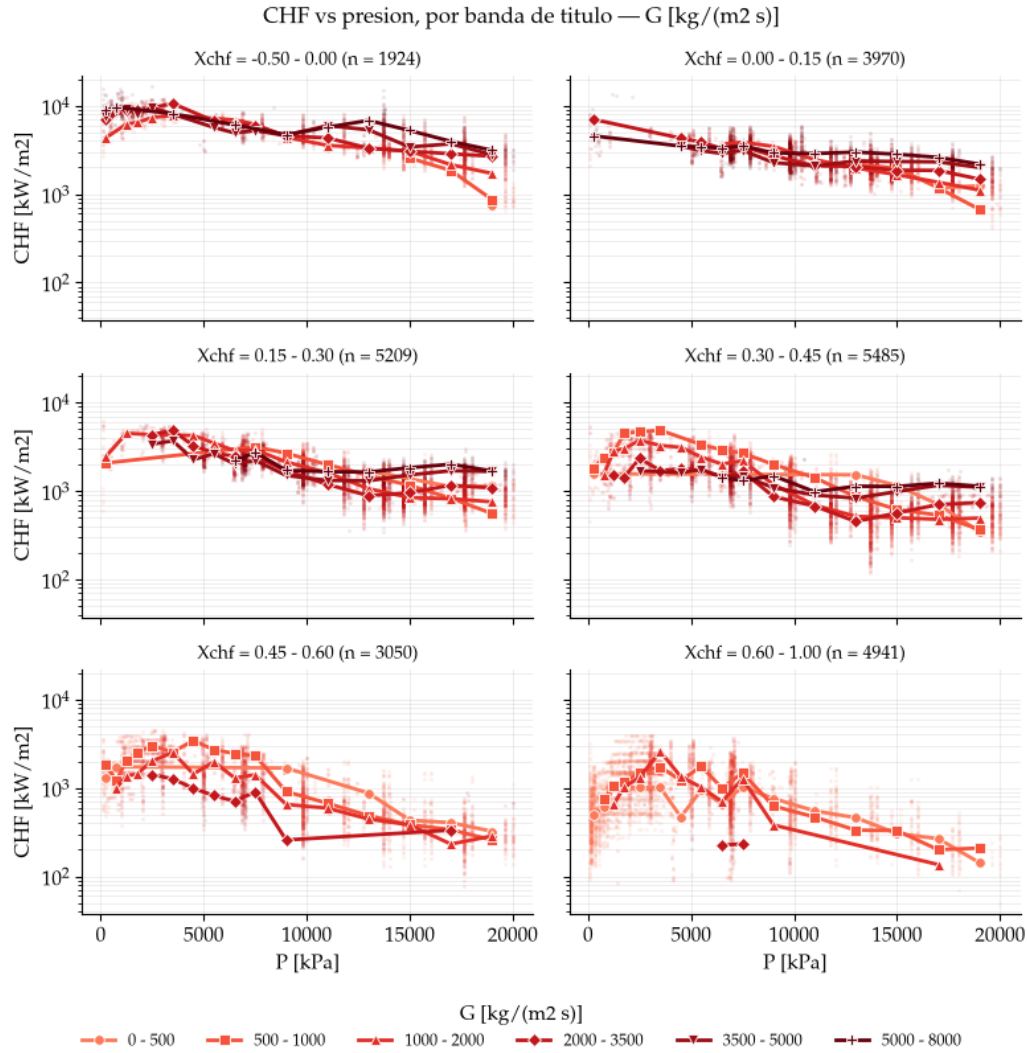
FIGURA 3.9. Tendencia del CHF con la presión, para los datos de los ensayos en un tubo recopilados por Groeneveld [27, 9].
