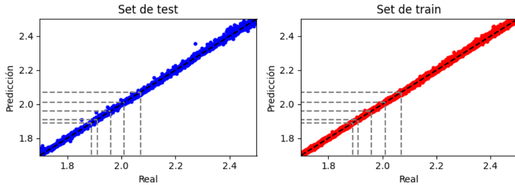
(B) Resultados preliminares de estimación de DNBR por DNN.
