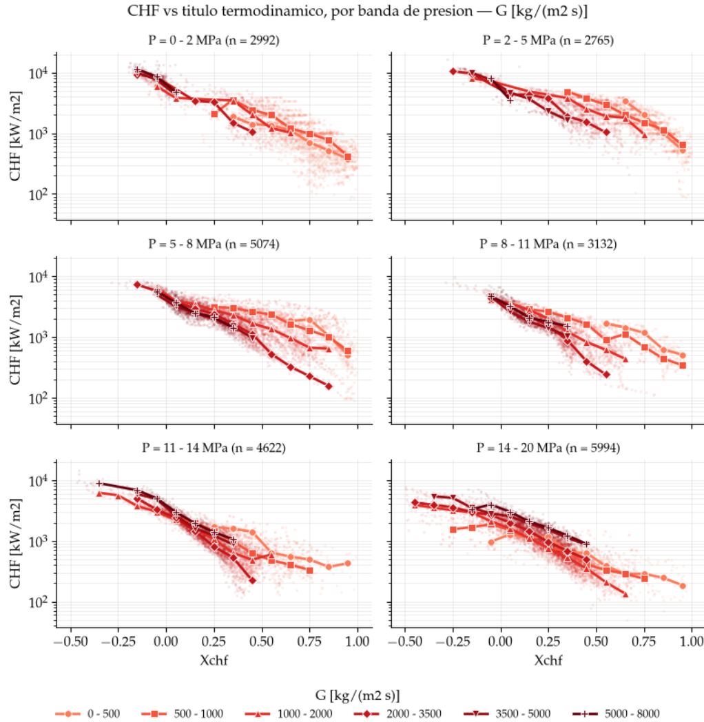
FIGURA 3.8. Tendencia del CHF con el título termodinámico, para los datos de los ensayos en un tubo recopilados por Groeneveld [27, 9].
