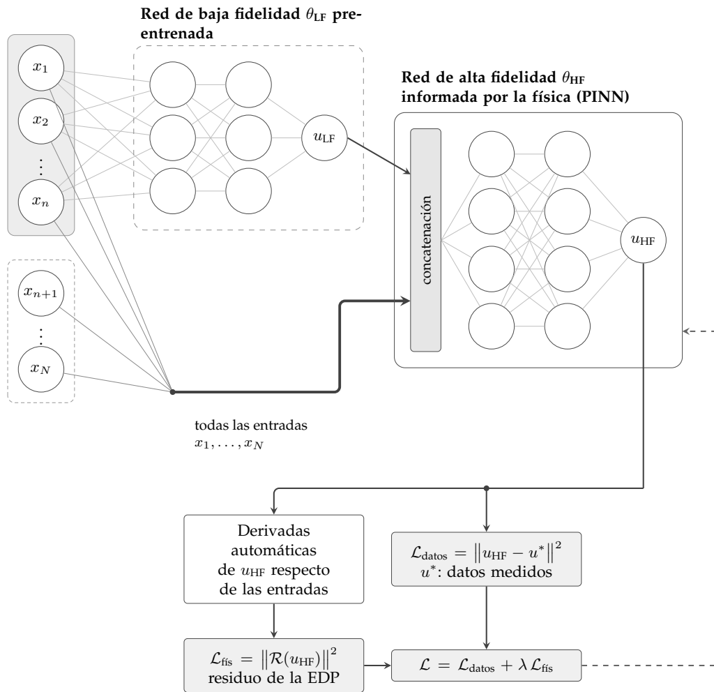
FIGURA 3.5. Esquema de la arquitectura de red neuronal de multifidelidad informada por física.
