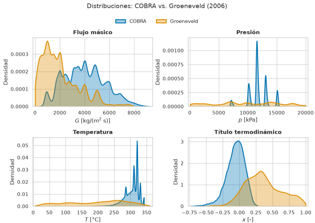
FIGURA 3.4. Comparativa de distribuciones de datos de flujo másico, presión, temperatura y título termodinámico entre ensayos de un tubo de Groeneveld y todos los puntos de los ensayos numéricos con COBRA3-CP.
