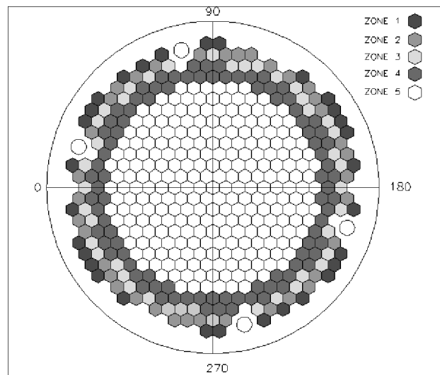
FIGURA 1.2. Esquematización de los canales refrigerantes en el núcleo de la CNA-UII y las 5 zonas hidráulicas. [1]
