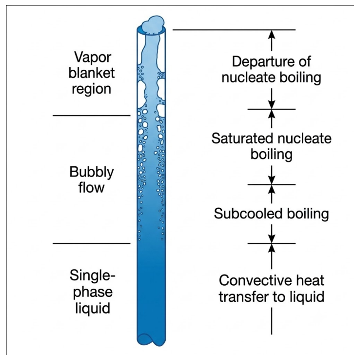
FIGURA 1.4. Esquematzación del Apartamiento de la Ebullición Nucleada (DNB) en un tubo.
