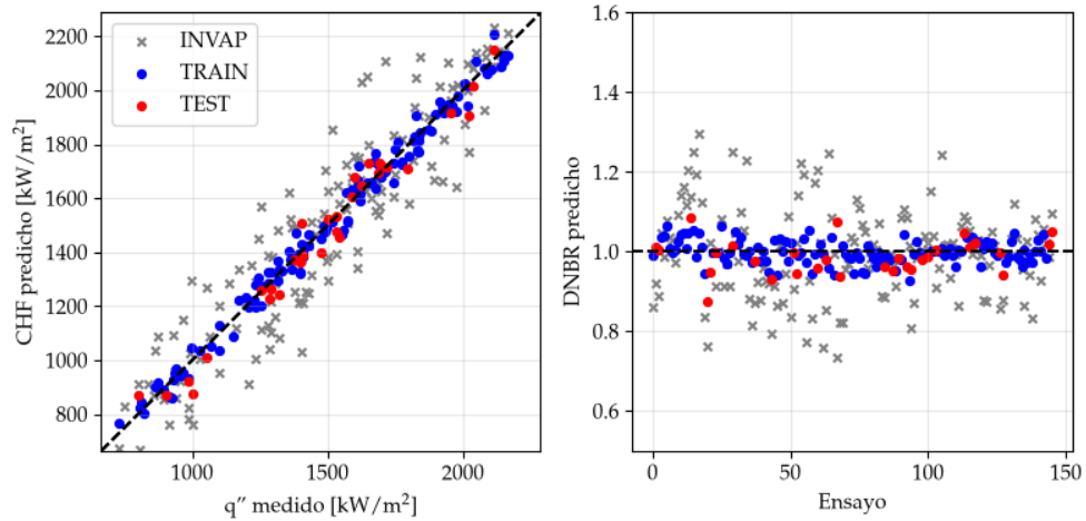
FIGURA 4.11. CHF predicho contra medido y DNBR por ensayo para modelo final MFP INN.
