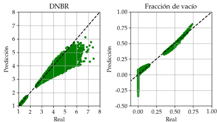
FIGURA B.2. Resultados de predicción de DNBR y fracción de vacío, para el conjunto excluido.
