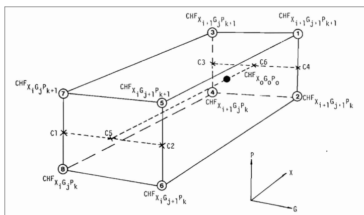
FIGURA A.1. Esquematización de interpolación en tres dimensiones en la LUT de Groeneveld 1 .
