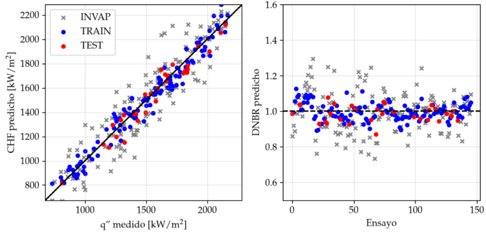
FIGURA 4.10. CHF predicho contra medido y DNBR por ensayo para modelo final MFDNN.
