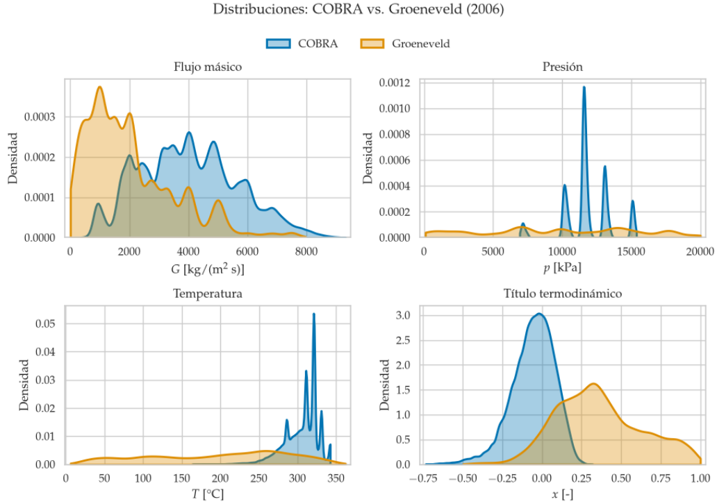
FIGURA 3.5. Comparativa de distribuciones de datos de flujo másico, presión, temperatura y título termodinámico entre ensayos en un tubo de Groeneveld y todos los puntos de los ensayos numéricos con COBRA3-CP.
