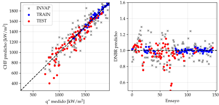
FIGURA 4.8. CHF predicho contra medido y DNBR por ensayo para variante E de MFP INN.
