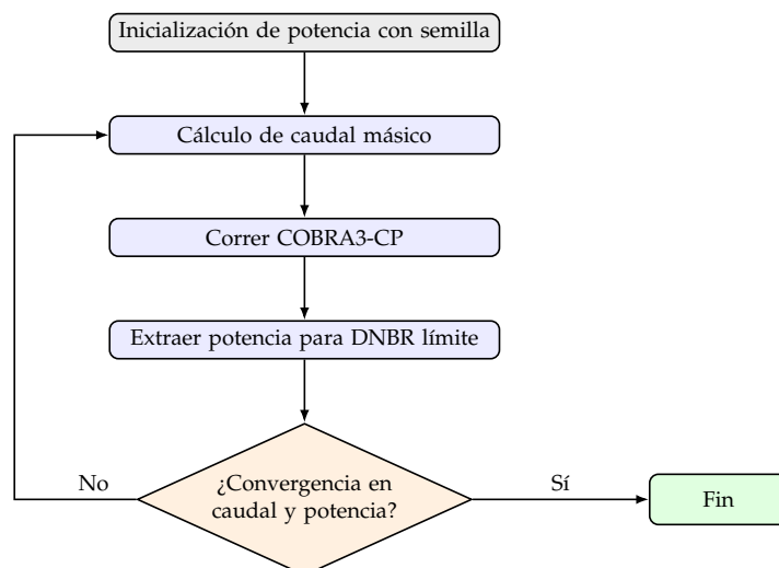
FIGURA 2.1. Esquema del lazo de cálculo iterativo de la PLC por DNBR con COBRA3-CP.
