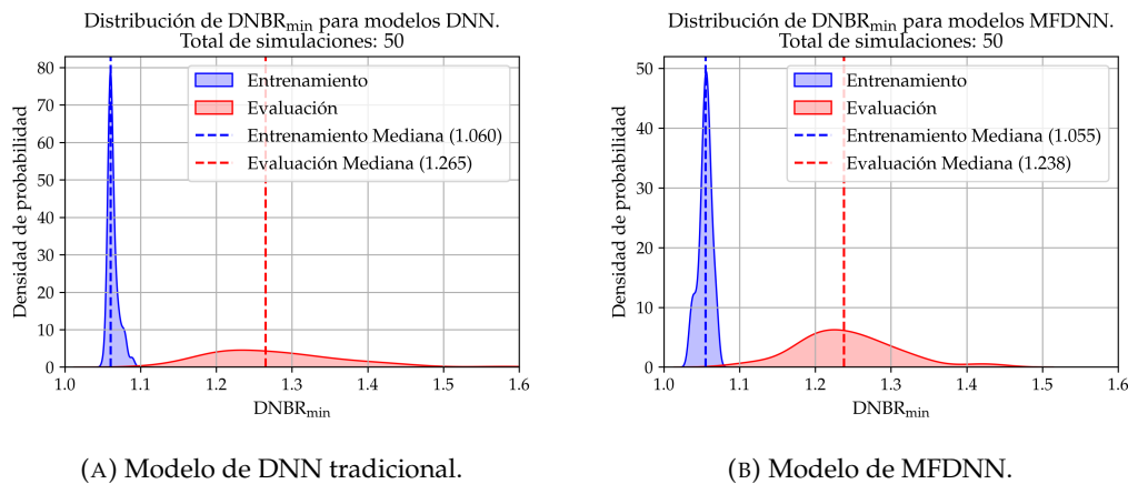
FIGURA 4.6. Distribución de probabilidad de \text{DNBR}_{\min} para N = 50 modelos entrenados de cada tipo.
