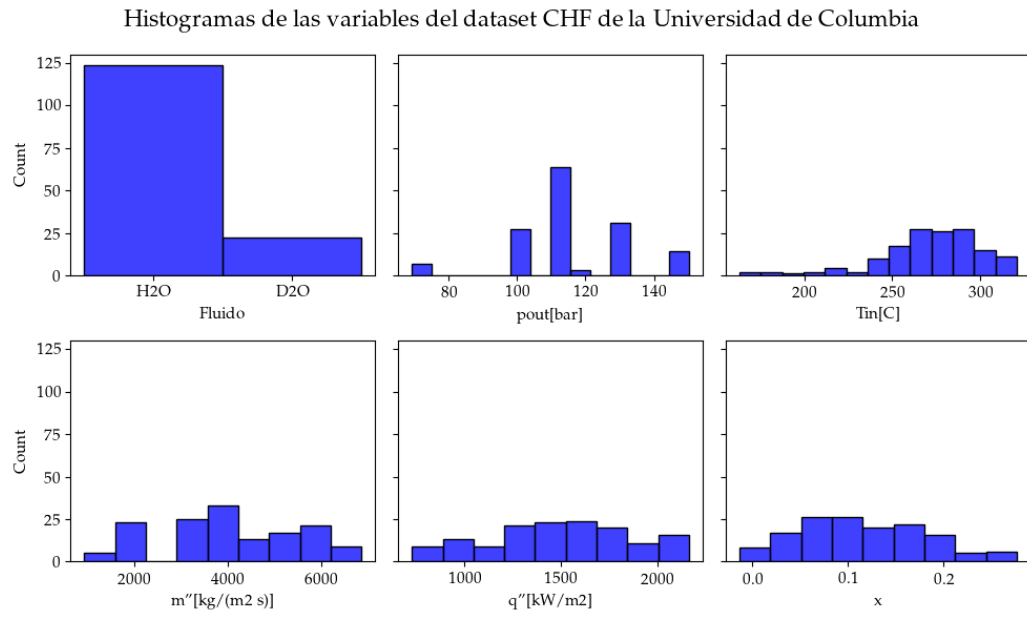
FIGURA 2.4. Histogramas de las variables de los ensayos de CHF de la UC.
