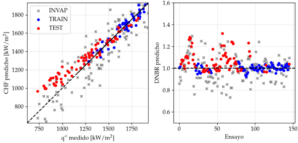
FIGURA C.14. CHF predicho contra medido y DNBR por ensayo, para MFDNN con variables de entrada expandidas.
