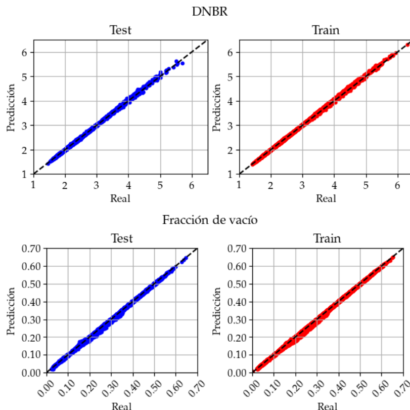
FIGURA 4.1. Resultados de predicción de DNBR y fracción de vacío, para los conjuntos de evaluación y entrenamiento.
