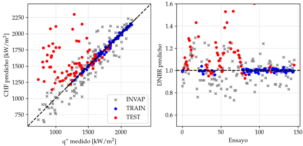
FIGURA C.15. CHF predicho contra medido y DNBR por ensayo, para variante E de MFPINN con variables de entrada expandidas.
