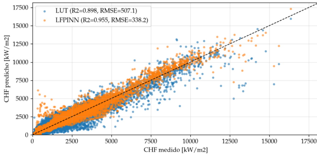
FIGURA 4.13. Predicción de CHF contra medido para LFPINN y LUT.
