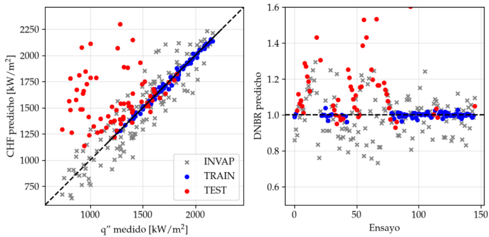
FIGURA C.15. CHF predicho contra medido y DNBR por ensayo, para variante E de MFPINN con variables de entrada expandidas.
