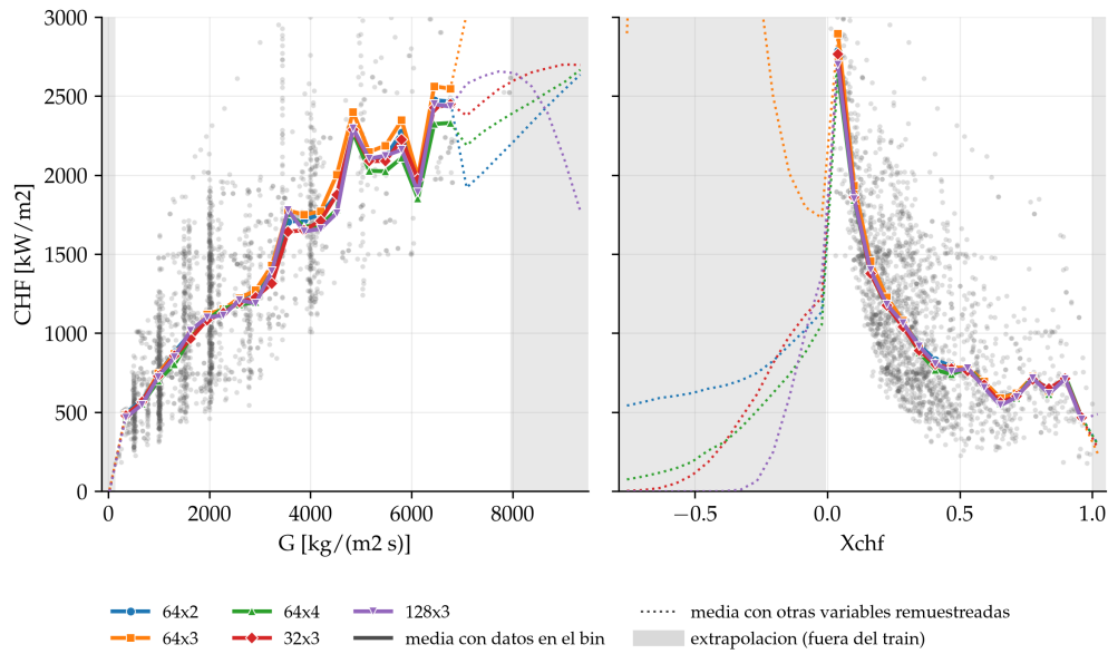
FIGURA C.2. Evaluación de la generalización de la LFDNN respecto del flujo másico y el título termodinámico.
