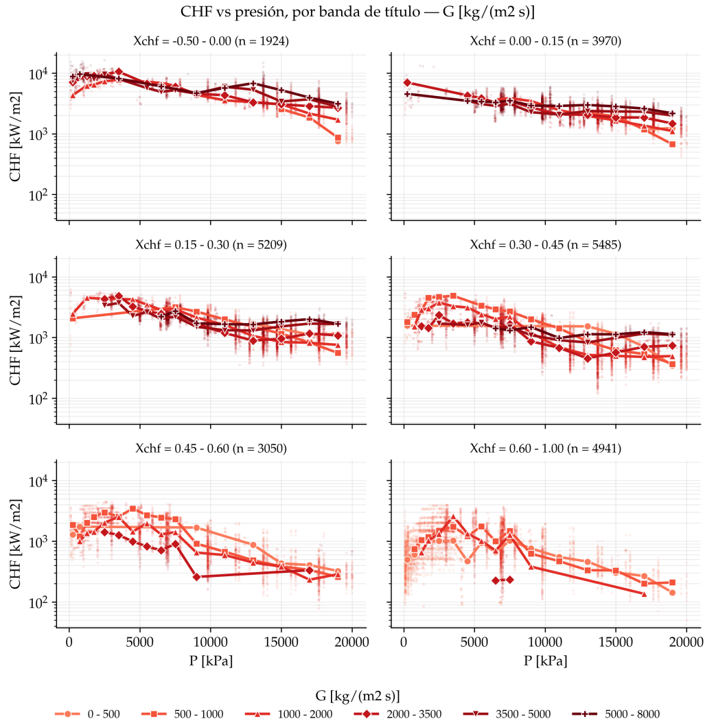
FIGURA 3.9. Tendencia del CHF con la presión, para los datos de los ensayos en un tubo recopilados por Groeneveld [1, 2].
