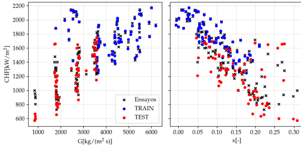
FIGURA C.10. Relación entre CHF predicho y flujo másico y título termodinámico para variante A de MFP INN.
