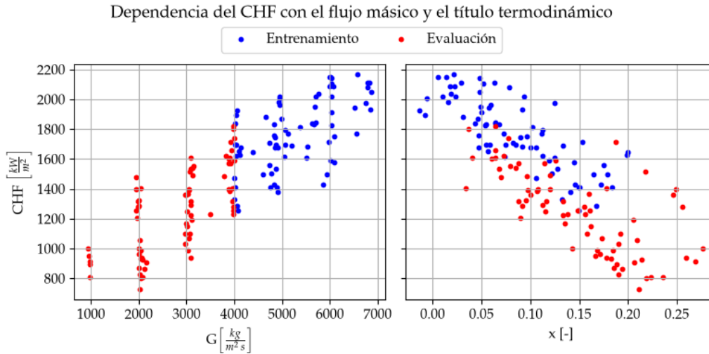
FIGURA 4.5. División de los datos de CHF de la UC en entrenamiento y evaluación, según flujo másico. Los ejes de flujo másico y título termodinámico corresponden a los valores promedio de la sección de ensayo a la salida.
