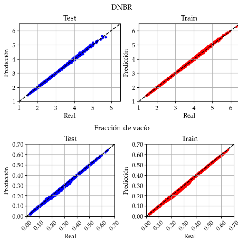
FIGURA 4.1. Resultados de predicción de DNBR y fracción de vacío, para los conjuntos de test y train.
