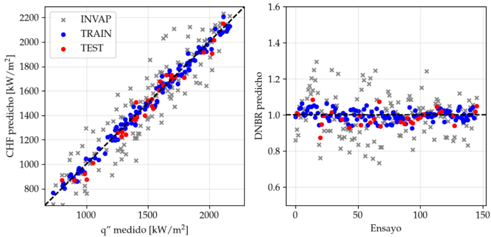
FIGURA 4.11. CHF predicho contra real y DNBR por ensayo para modelo final MFP INN.
