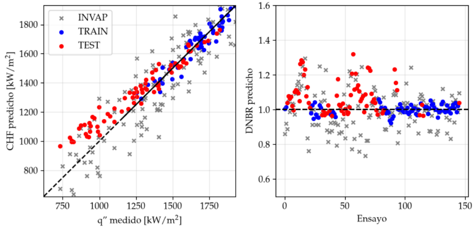
FIGURA C.14. CHF predicho contra real y DNBR por ensayo, para MFDNN con variables de entrada expandidas.
