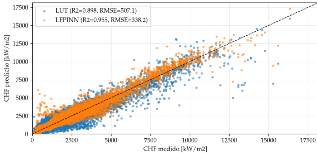
FIGURA C.6. Predicción de CHF contra medido para LFPINN y LUT.
