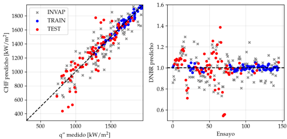
FIGURA C.8. CHF predicho contra medido y DNBR por ensayo para variante B de MFP INN.
