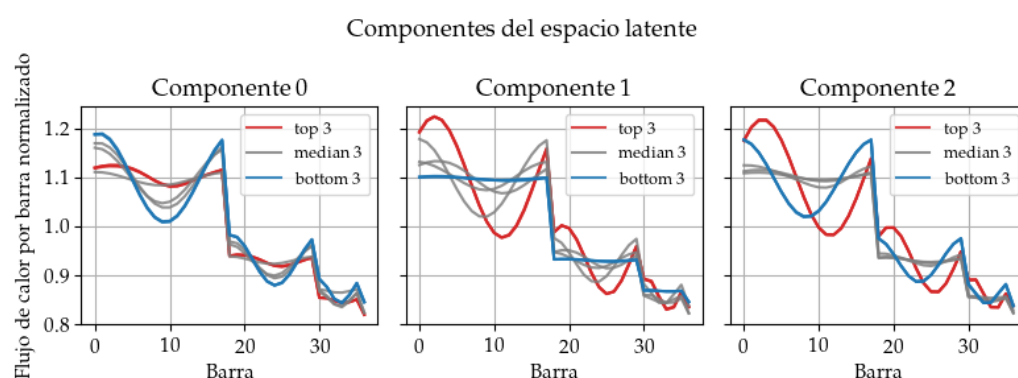
FIGURA 4.4. Gráficos de perfiles radiales con valores más altos, medianos y bajos de cada componente del espacio latente.
