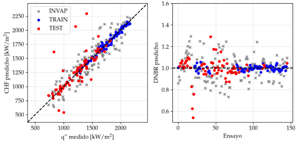
FIGURA C.9. CHF predicho contra medido y DNBR por ensayo para variante D de MFP INN.
