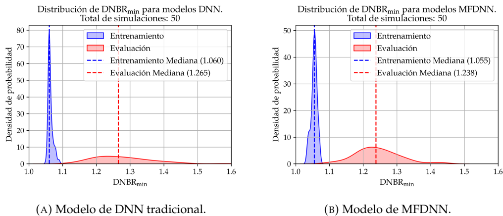
FIGURA 4.6. Distribución de probabilidad de DNBR_{min} para N = 50 modelos entrenados de cada tipo.
