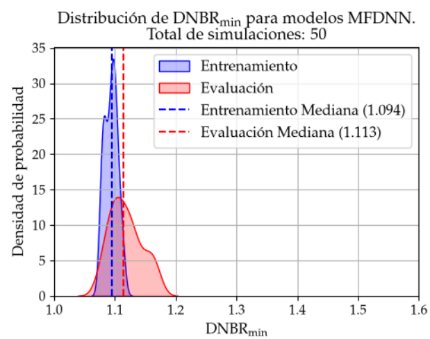
FIGURA C.16. Distribución de densidad de probabilidad de \text{DNBR}_{\min} para 50 modelos MFDNN entrenados.
