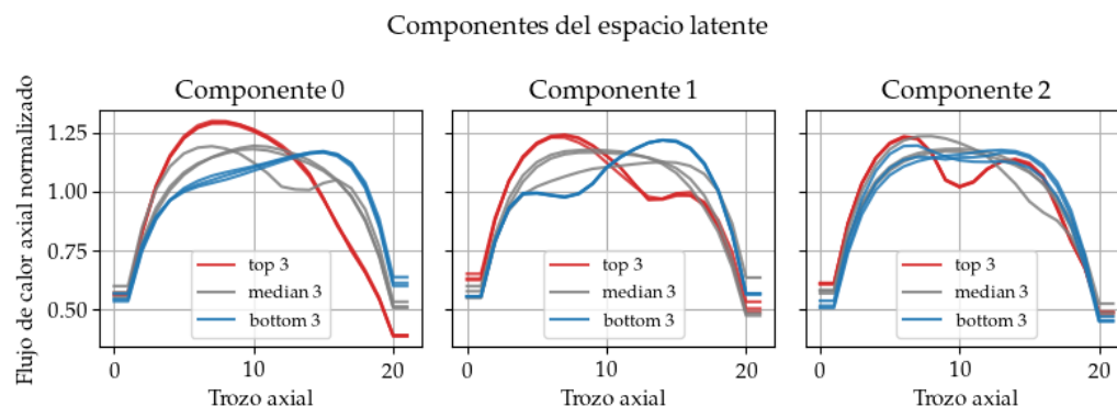
FIGURA 4.3. Gráficos de perfiles axiales con valores más altos, medianos y bajos de cada componente del espacio latente.
