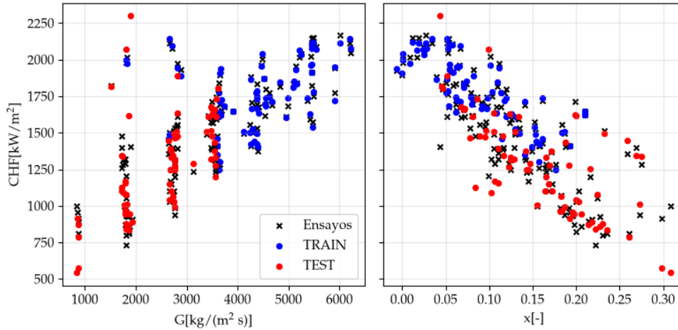
FIGURA C.12. Relación entre CHF predicho y flujo másico y título termodinámico para variante D de MFP INN.
