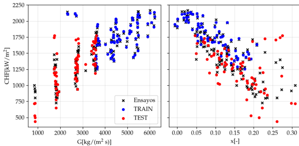
FIGURA C.11. Relación entre CHF predicho y flujo másico y título termodinámico para variante B de MFP INN.
