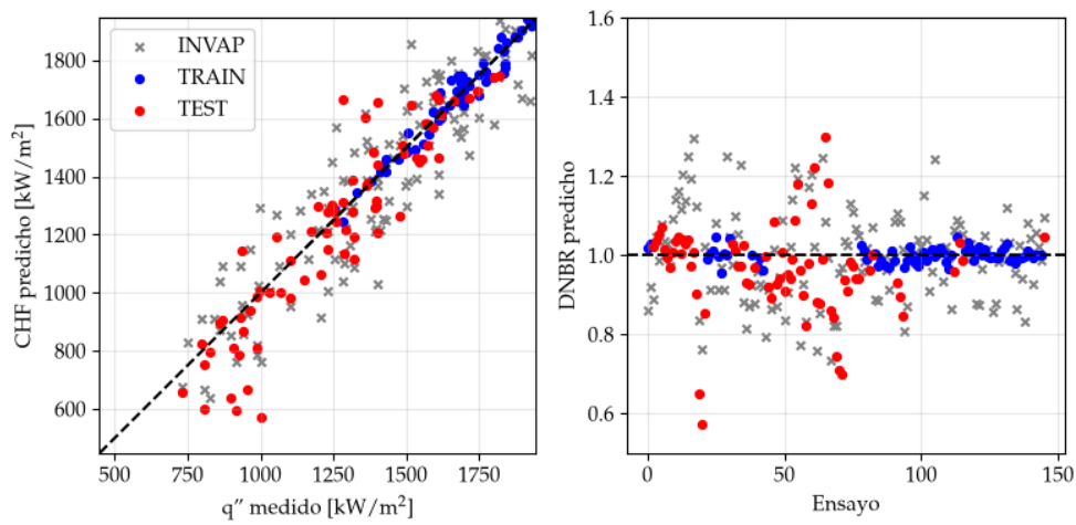
FIGURA C.7. CHF predicho contra medido y DNBR por ensayo para variante A de MFP INN.
