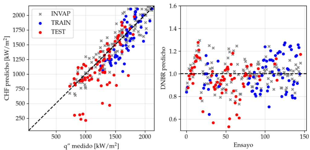
FIGURA C.5. Predicción de CHF contra medido y DNBR para cada ensayo, para modelo LFPINN con \lambda = 0,1 .
