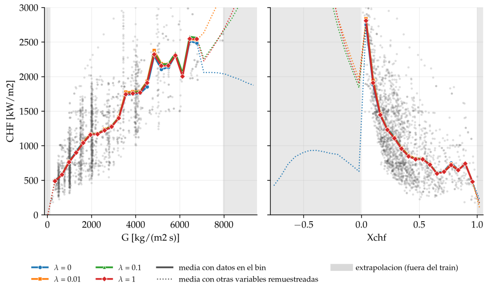
FIGURA C.4. Evaluación de la generalización de la LFPINN respecto del flujo másico y el título termodinámico, según \lambda .
