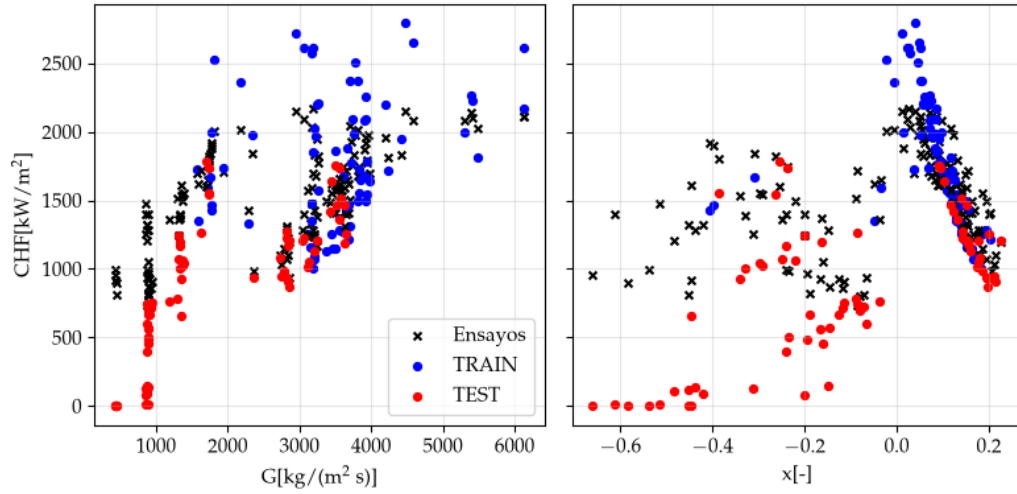
FIGURA C.1. Relación del CHF predicho con el flujo másico y el título, según el punto predicho por el modelo LFDNN\#4 . TRAIN y TEST son los conjuntos de entrenamiento y evaluación correspondientes a la HFDNN , divididos tal que en evaluación se tienen los ensayos de menor flujo másico.
