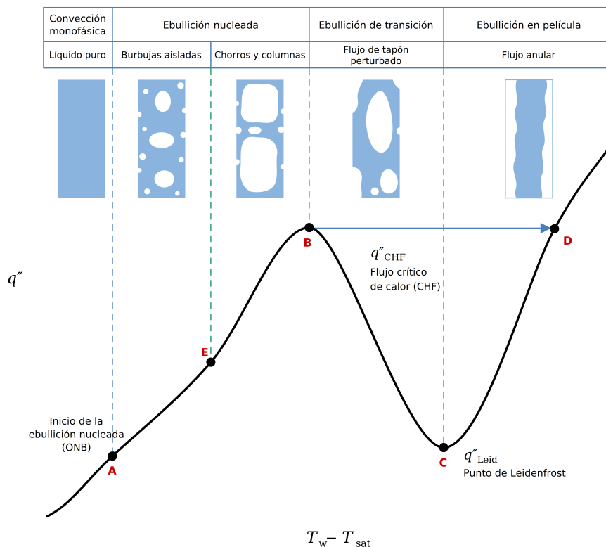
FIGURA 1.3. Curva de Nukiyama 3 .
