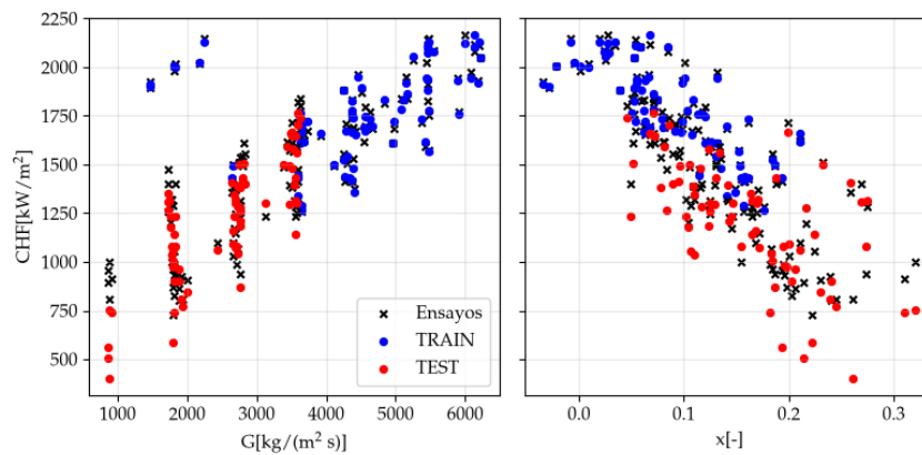
FIGURA 4.9. Relación entre CHF predicho y flujo másico y título termodinámico para variante E de MFP INN.
