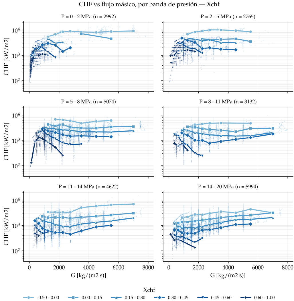
FIGURA 3.7. Tendencia del CHF con el flujo másico, para los datos de los ensayos en un tubo recopilados por Groeneveld [1, 2].
