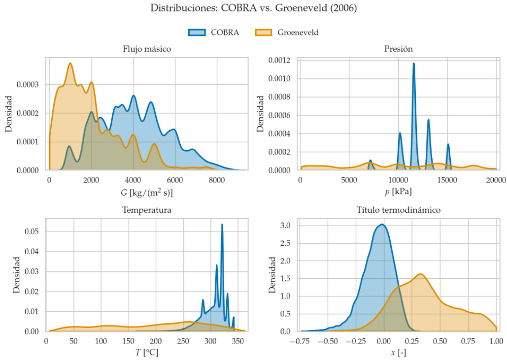
FIGURA 3.5. Comparativa de distribuciones de datos de flujo máscico, presión, temperatura y título termodinámico entre ensayos de un tubo de Groeneveld y todos los puntos de los ensayos numéricos con COBRA3-CP.
