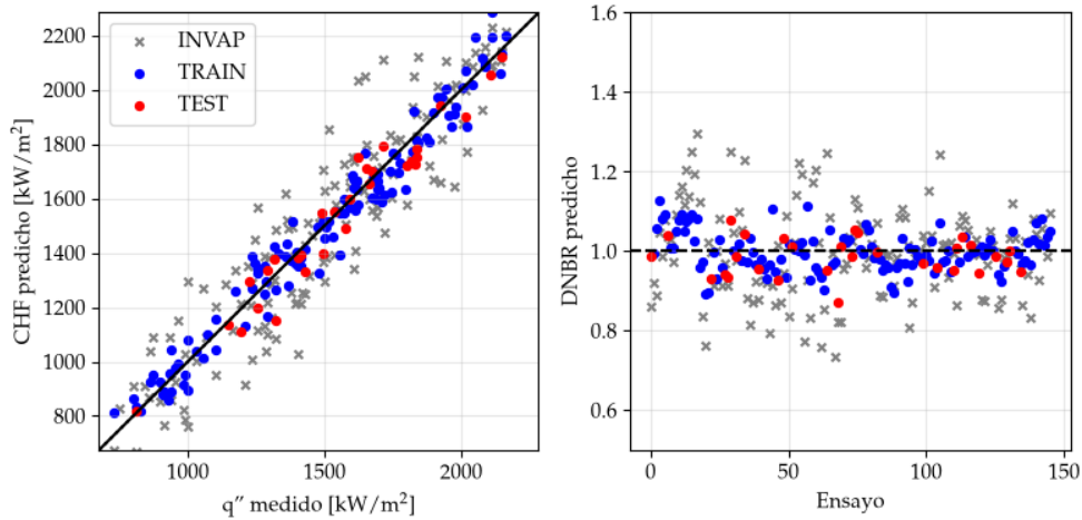
FIGURA 4.10. CHF predicho contra real y DNBR por ensayo para modelo final MFDNN.
