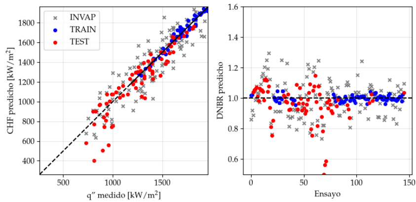
FIGURA 4.8. CHF predicho contra medido y DNBR por ensayo para variante E de MFP INN.
