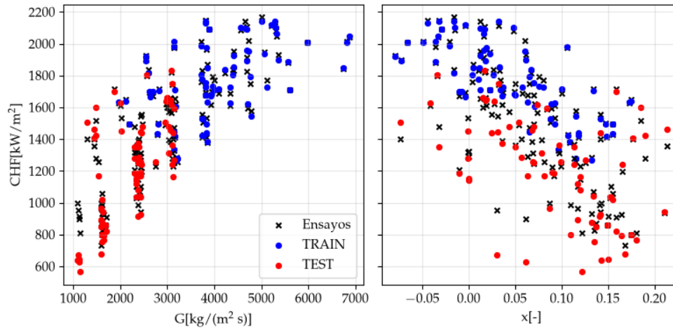
FIGURA C.13. Relación de CHF con el flujo másico y el título termodinámico para variante D de MFPINN, con variables de entrada expandidas.
