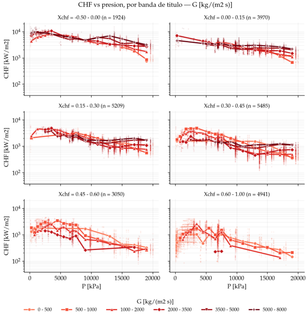
FIGURA 3.9. Tendencia del CHF con la presión, para los datos de los ensayos en un tubo recopilados por Groeneveld [27, 9].
