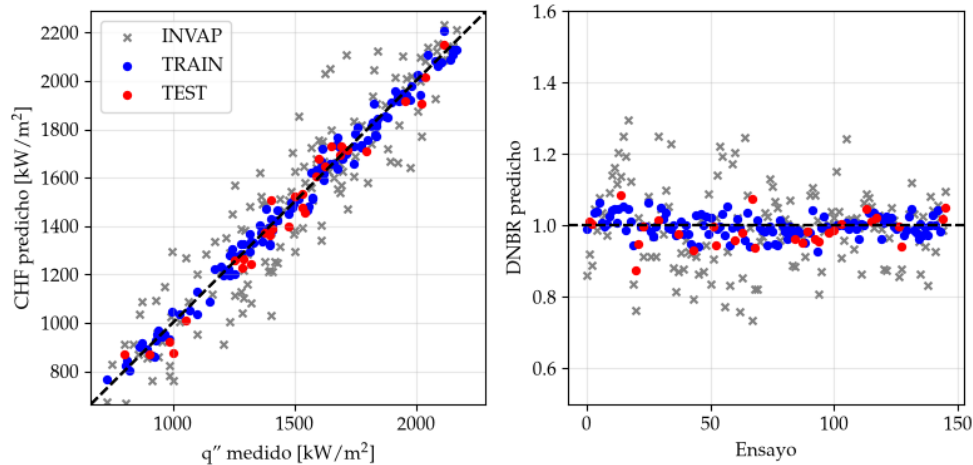
FIGURA 4.11. CHF predicho contra real y DNB por ensayo para modelo final MFP INN.
