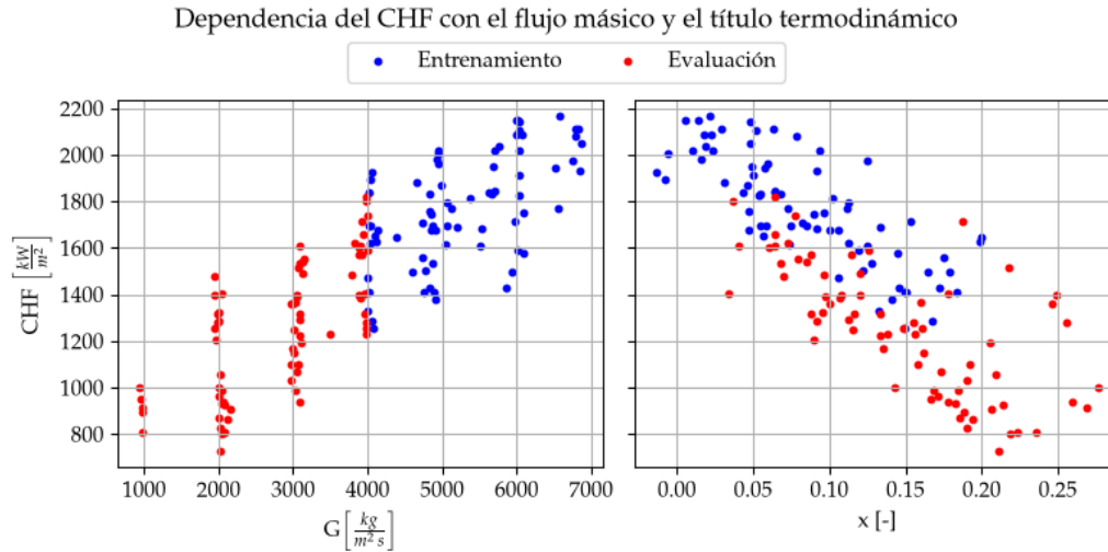
FIGURA 4.5. División de los datos de CHF de la Universidad de Columbia en entrenamiento y evaluación, según flujo másico. Los ejes de flujo másico y título termodinámico corresponden a los valores promedio de la sección de ensayo a la salida.
