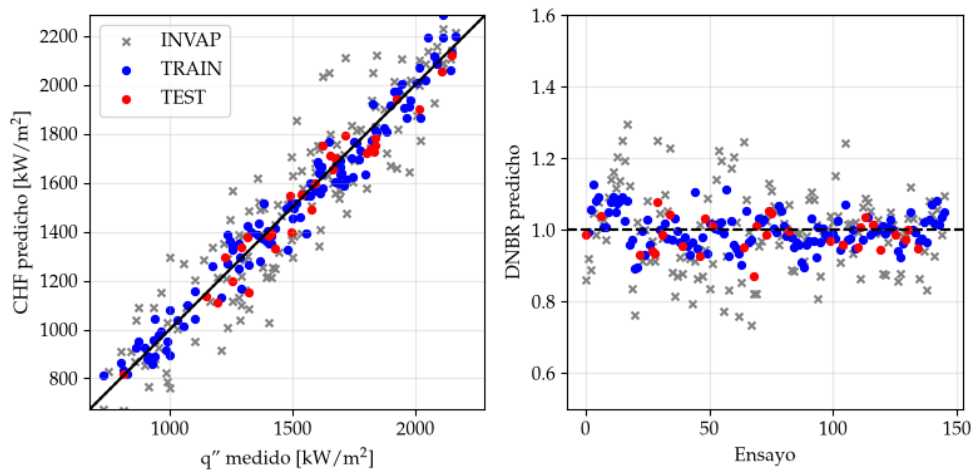
FIGURA 4.10. CHF predicho contra real y DNBR por ensayo para modelo final MFDNN .
