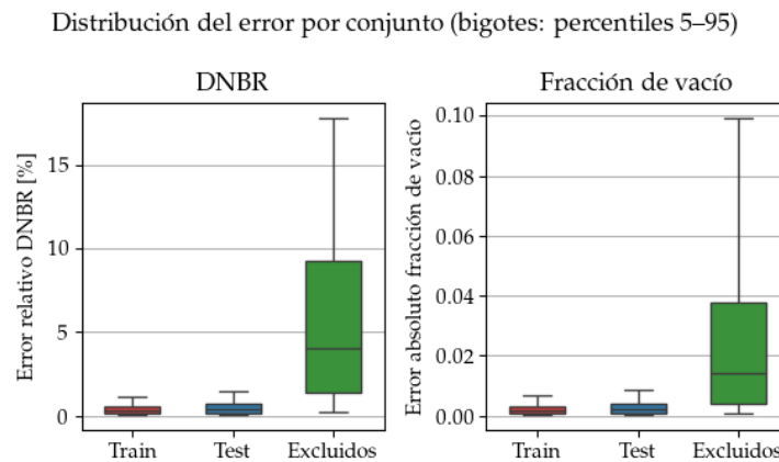
FIGURA B.3. Distribución del error para cada objetivo, por conjunto de datos.
