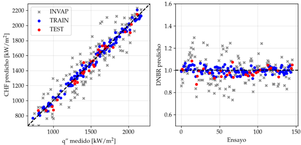
FIGURA 4.29. CHF predicho contra real y DNBR por ensayo para modelo final MFPINN.
