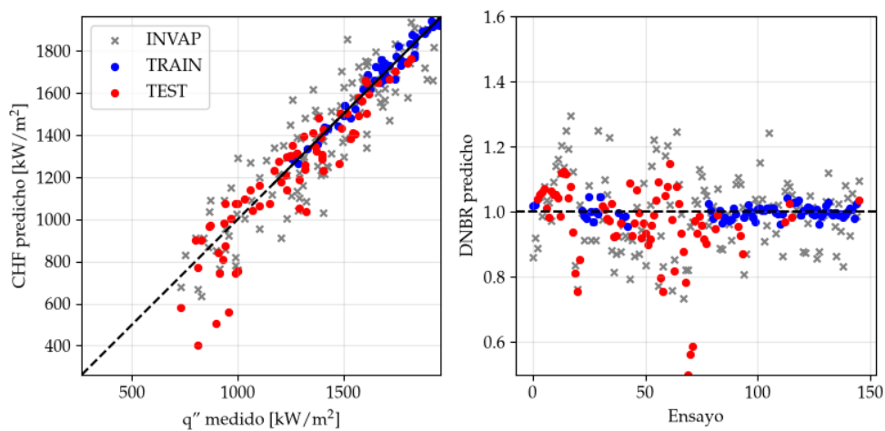
FIGURA 4.20. CHF predicho contra medido y DNBR por ensayo para variante E de MFP INN.
