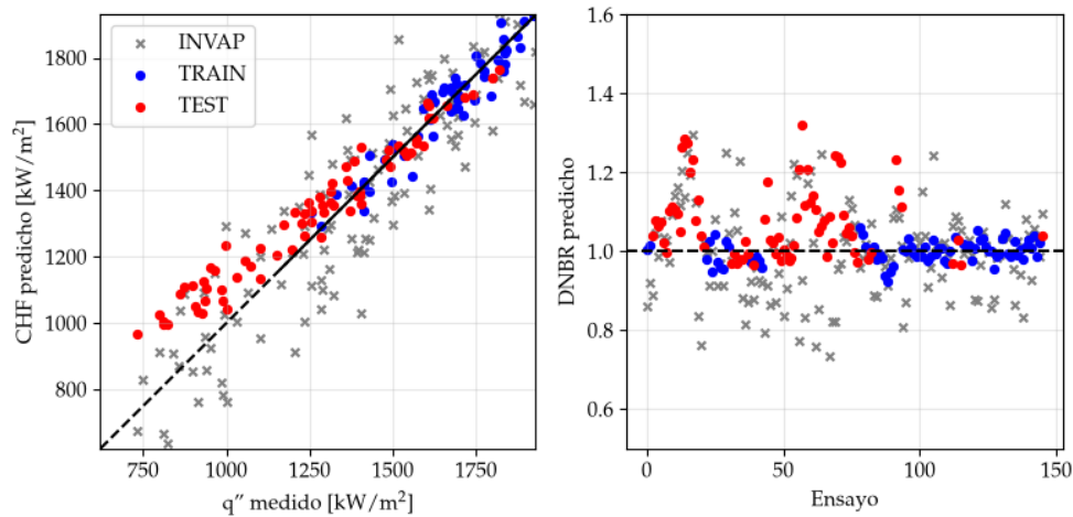
FIGURA 4.25. CHF predicho contra real y DNBR por ensayo, para MFDNN con variables de entrada expandidas.
