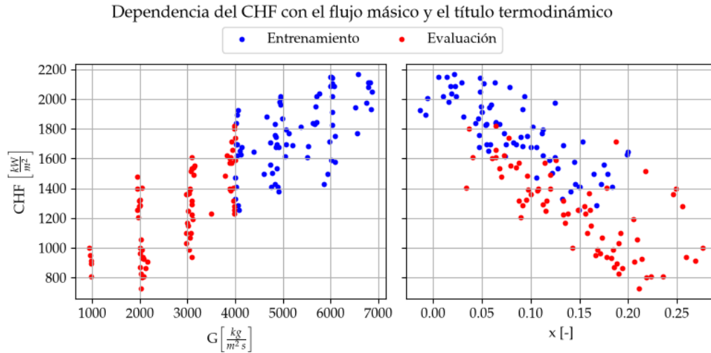
FIGURA 4.14. División de los datos de CHF de la Universidad de Columbia en entrenamiento y evaluación, según flujo másico. Los ejes de flujo másico y título termodinámico corresponden a los valores promedio de la sección de ensayo a la salida.
