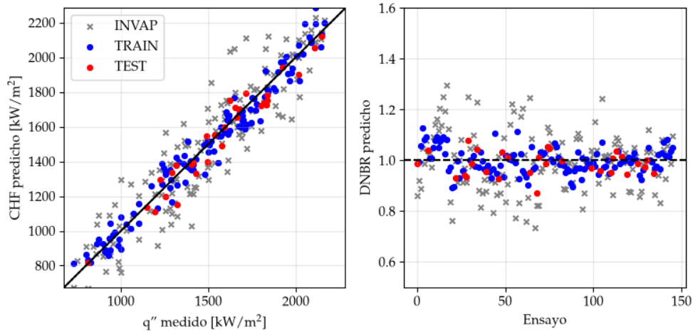
FIGURA 4.28. CHF predicho contra real y DNBR por ensayo para modelo final MFDNN.
