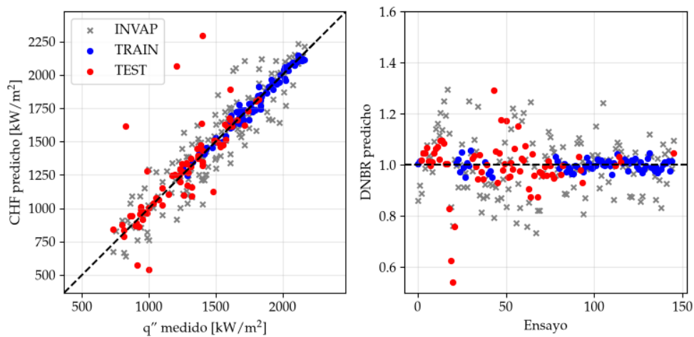
FIGURA 4.19. CHF predicho contra medido y DNBR por ensayo para variante D de MFP INN.
