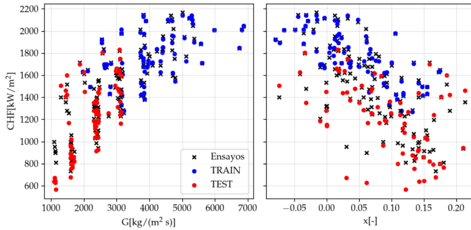
FIGURA 4.24. Relación de CHF con el flujo másico y el título termodinámico para variante D de MFP INN, con variables de entrada expandidas.
