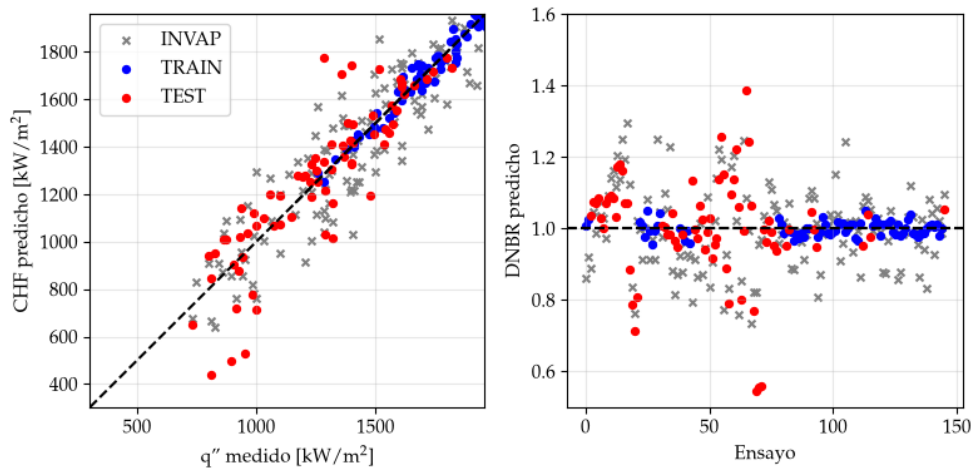
FIGURA 4.18. CHF predicho contra medido y DNBR por ensayo para variante B de MFP INN.
