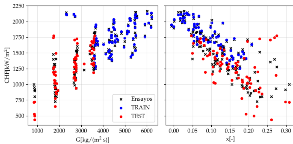
FIGURA 4.22. Relación entre CHF predicho y flujo másico y título termodinámico para variante B de MFP INN.
