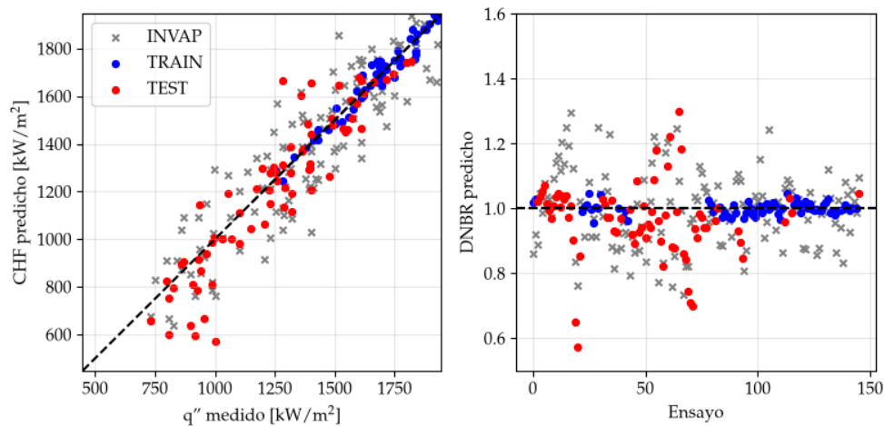
FIGURA 4.17. CHF predicho contra medido y DNBR por ensayo para variante A de MFP INN.
