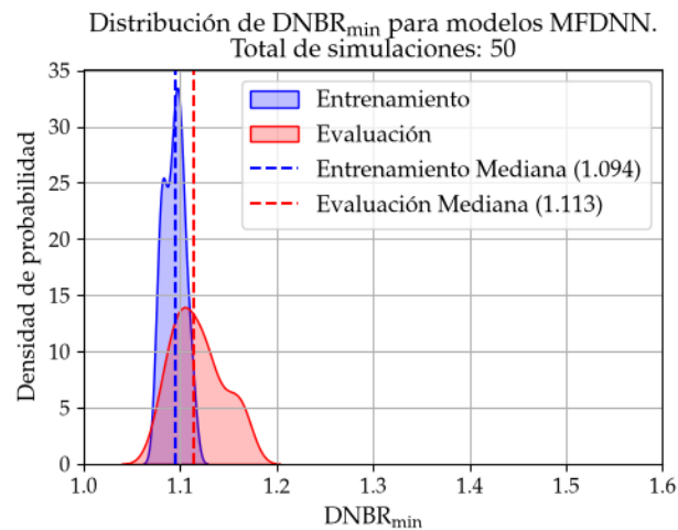
FIGURA 4.27. Distribución de densidad de probabilidad de DNBR_{min} para 50 modelos MFDNN entrenados.
