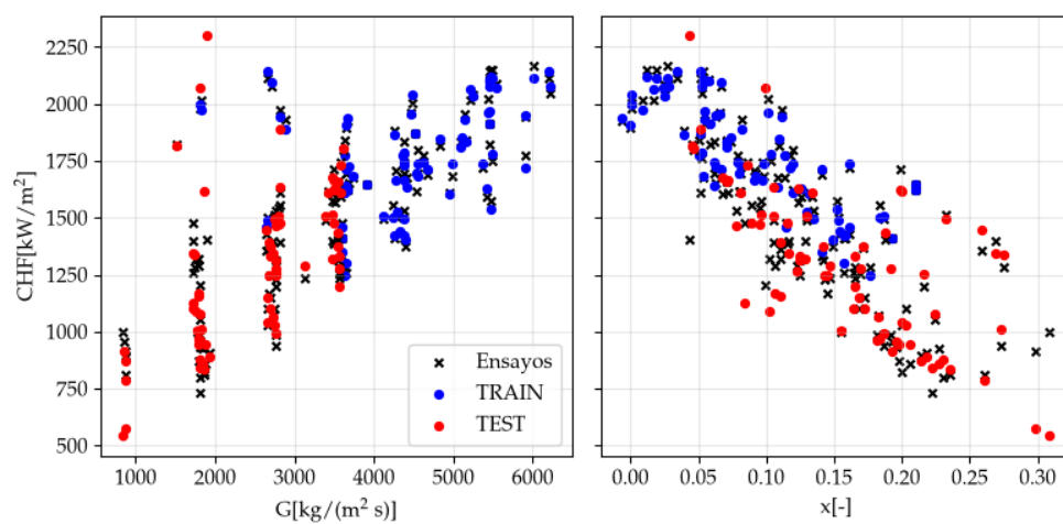
FIGURA 4.23. Relación entre CHF predicho y flujo másico y título termodinámico para variante D de MFP INN.
