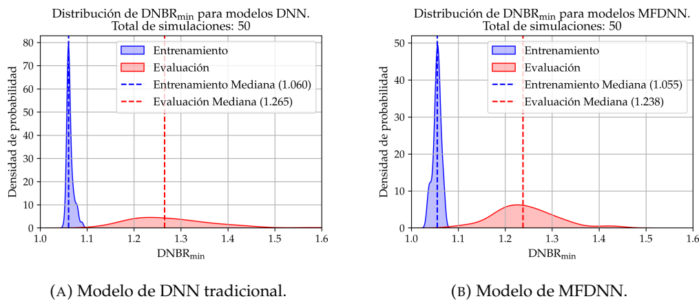
FIGURA 4.15. Distribución de probabilidad de \text{DNBR}_{\min} para N = 50 modelos entrenados de cada tipo.
