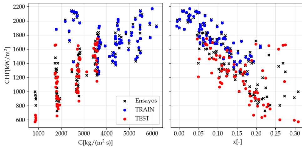
FIGURA 4.21. Relación entre CHF predicho y flujo másico y título termodinámico para variante A de MFP INN.
