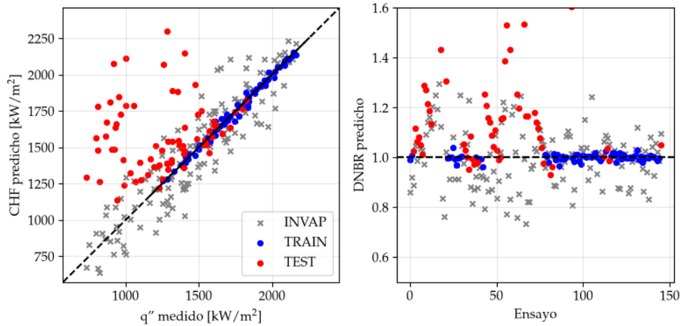
FIGURA 4.26. CHF predicho contra real y DNBR por ensayo, para variante E de MFP INN con variables de entrada expandidas.
