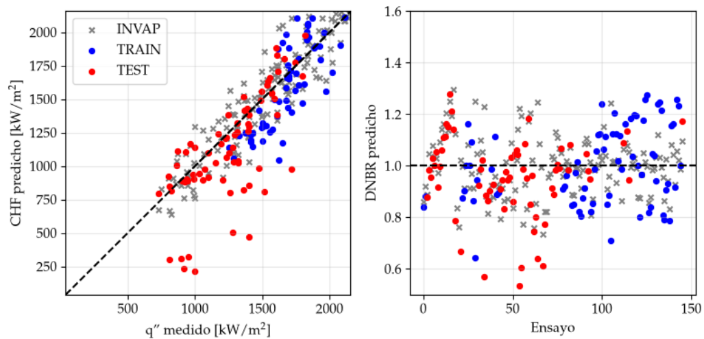
FIGURA 4.12. Predicción de CHF contra medido y DNBR para cada ensayo, para modelo LFP INN con \lambda = 0,1 .
