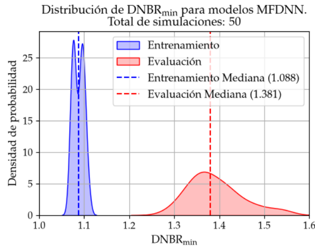
FIGURA 4.14. Distribución de probabilidad de \text{DNBR}_{\min} para N = 50 modelos entrenados de cada tipo.
