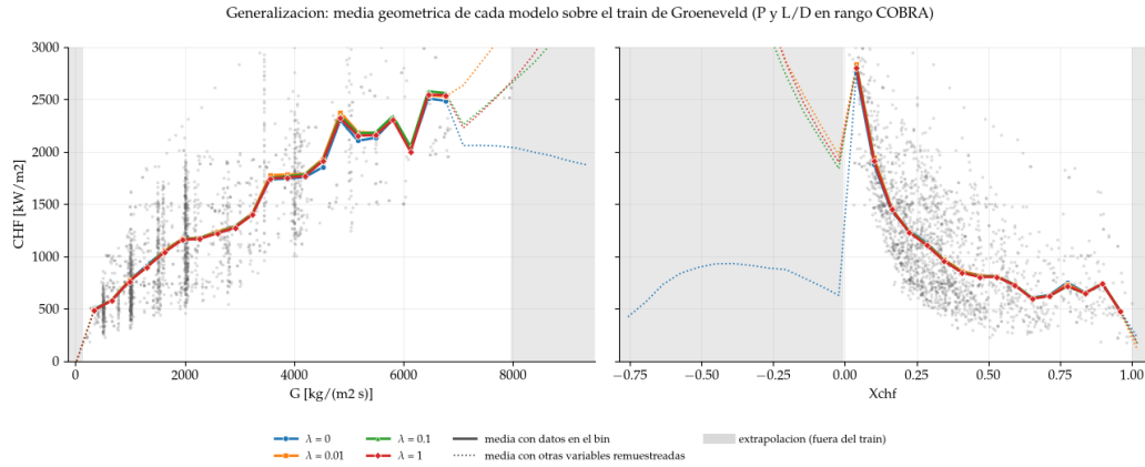
FIGURA 4.11. Evaluación de la generalización de la LFP INN respecto del flujo másico y el título termodinámico, según \lambda .
