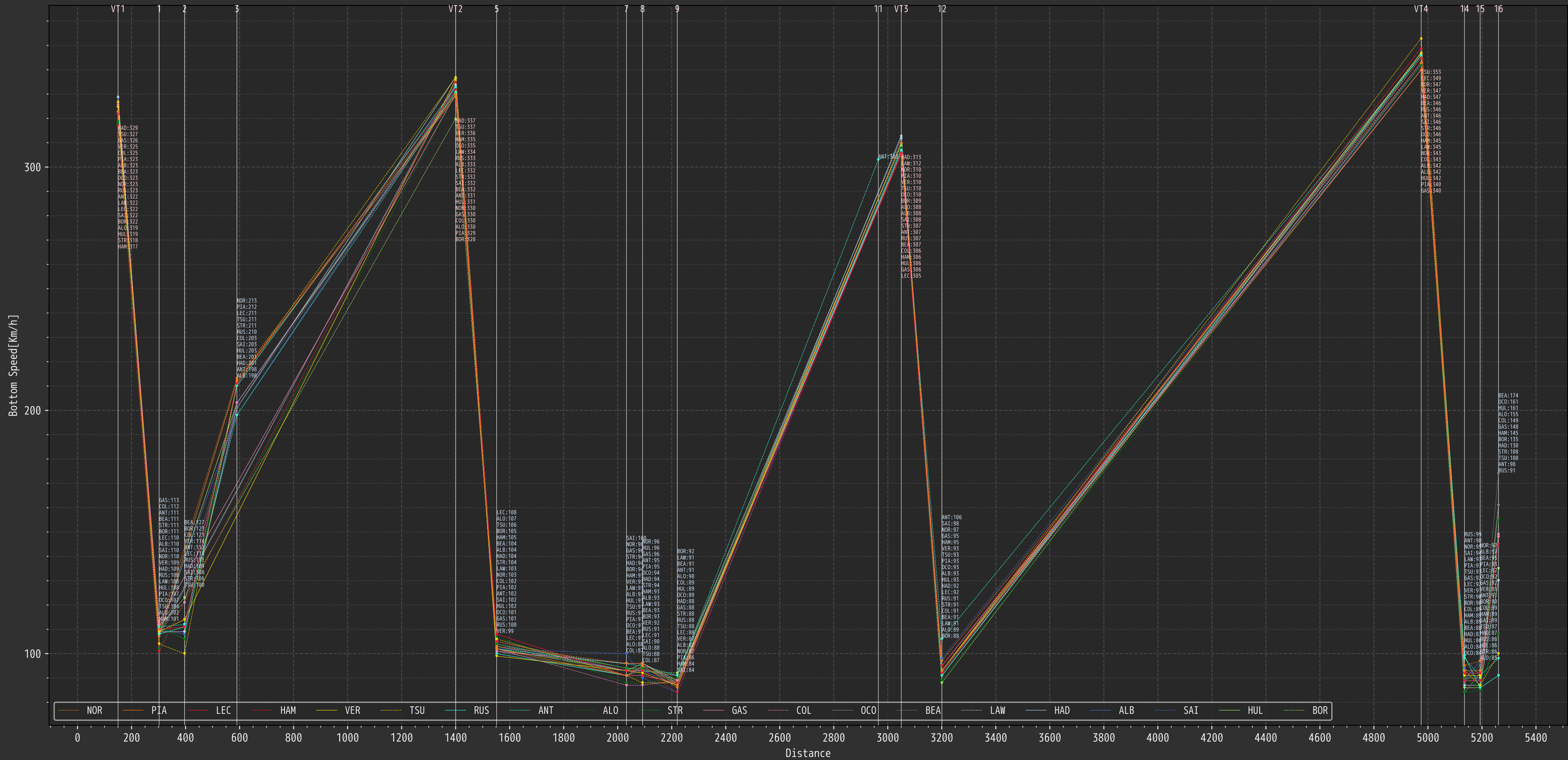
2025 Rd22 Las Vegas Grand Prix Practice 1 ファステストラップの各コーナーのボトムスピード(スロットル全開時を除く) + Virtual Speedtrap
