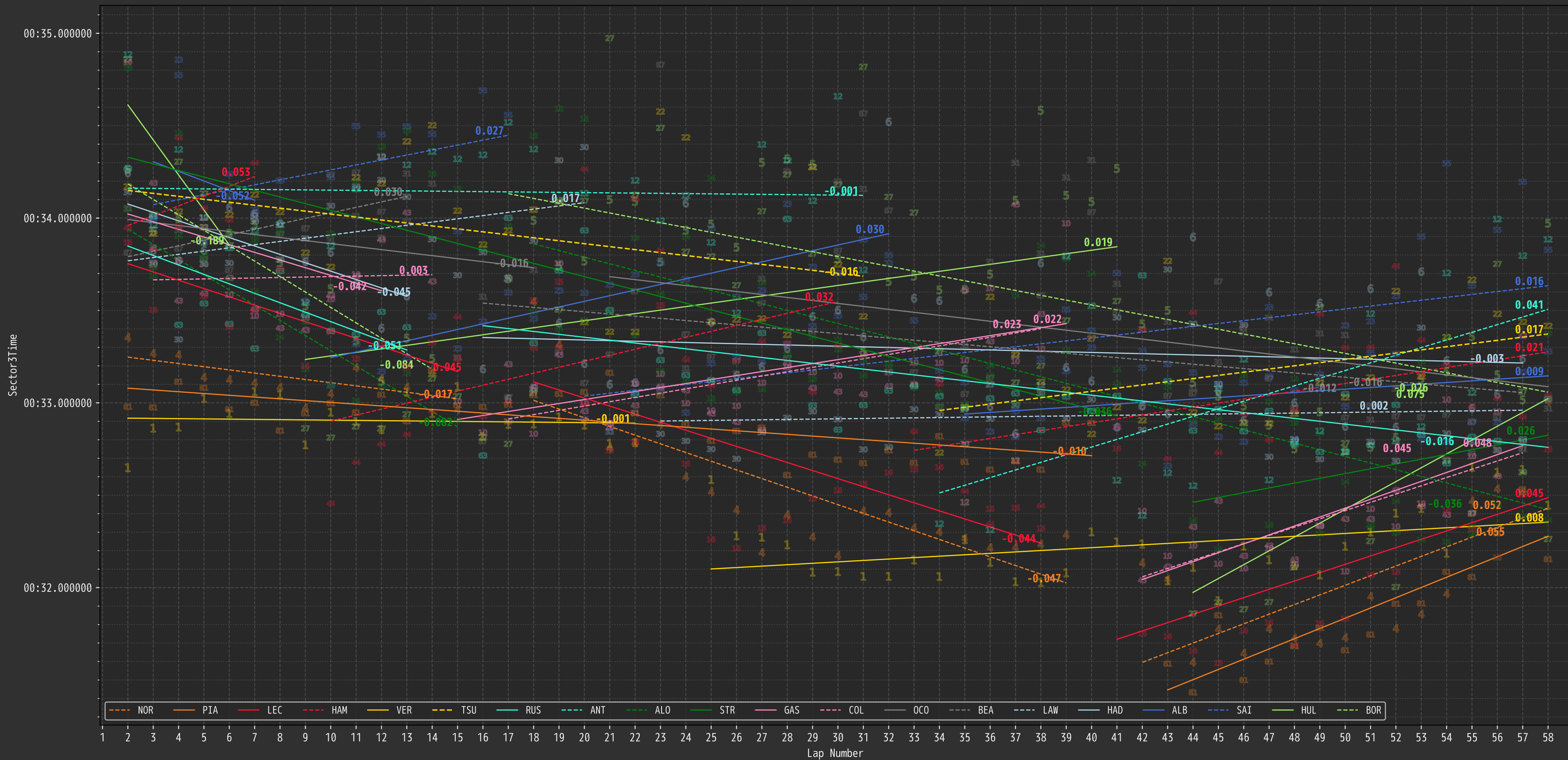
2025 Rd24 Abu Dhabi Grand Prix Race Sector3Timeの直線近似 直線近似 各ステントで0:31.000以上0:35.000以下の周回が3周以上の場合に算出
