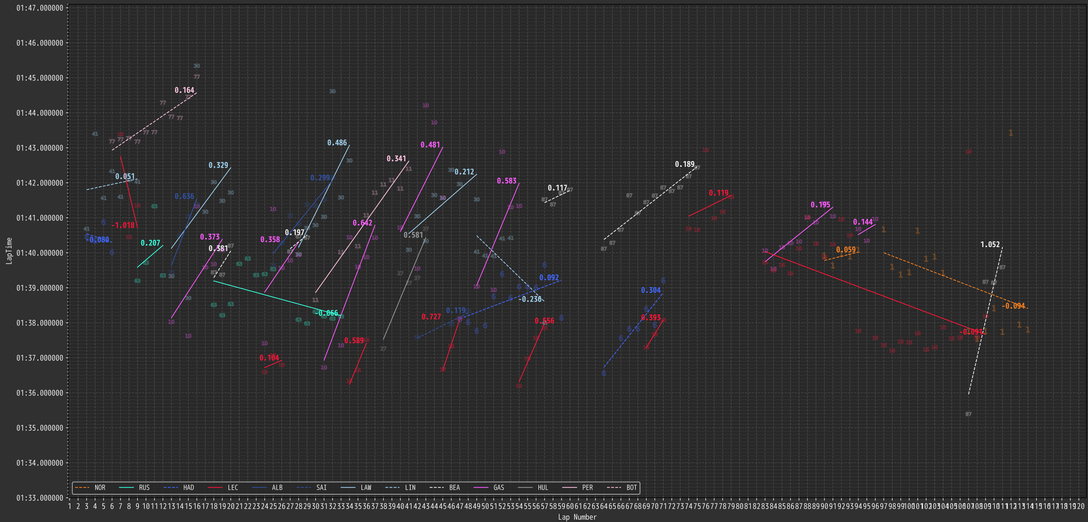
2026 Pre-Season Testing 1-2 S0FTタイヤのラップタイム直線近似 直線近似 各ステントで1:34.000以上1:46.000以下の周回が3周以上の場合に算出
