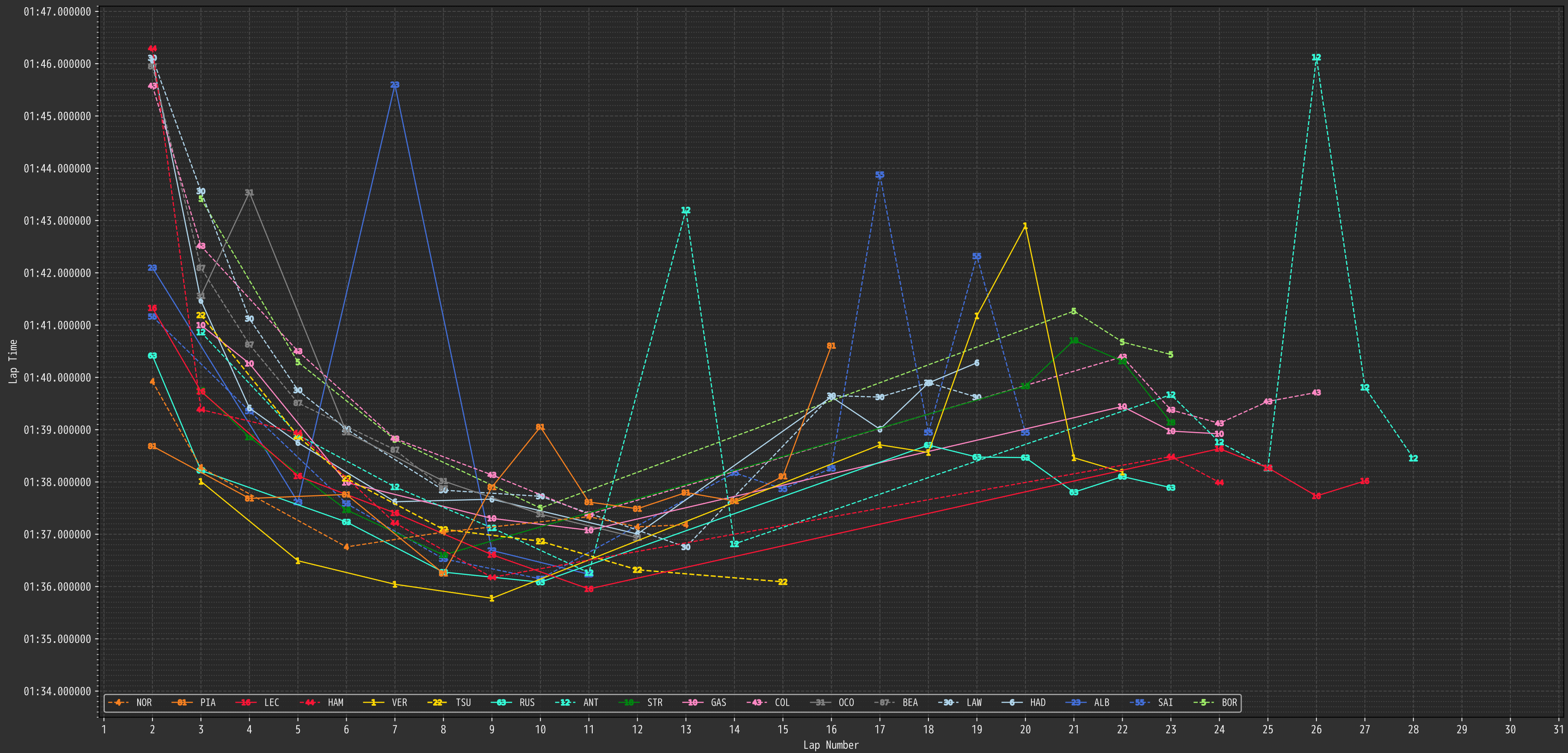
2025 Rd22 Las Vegas Grand Prix Practice1 MEDIUMタイヤのラップタイム (1:47.000までのタイムを抽出)
