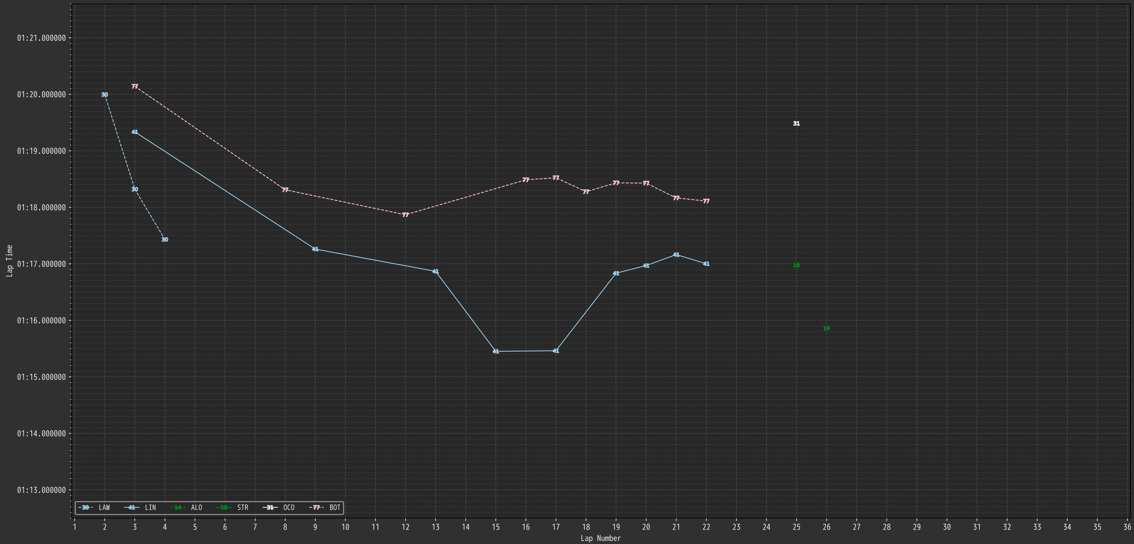
2026 Rd05 Canadian Grand Prix Practice 1 MEDIUMタイヤのラップタイム (1:21.500までのタイムを抽出)
