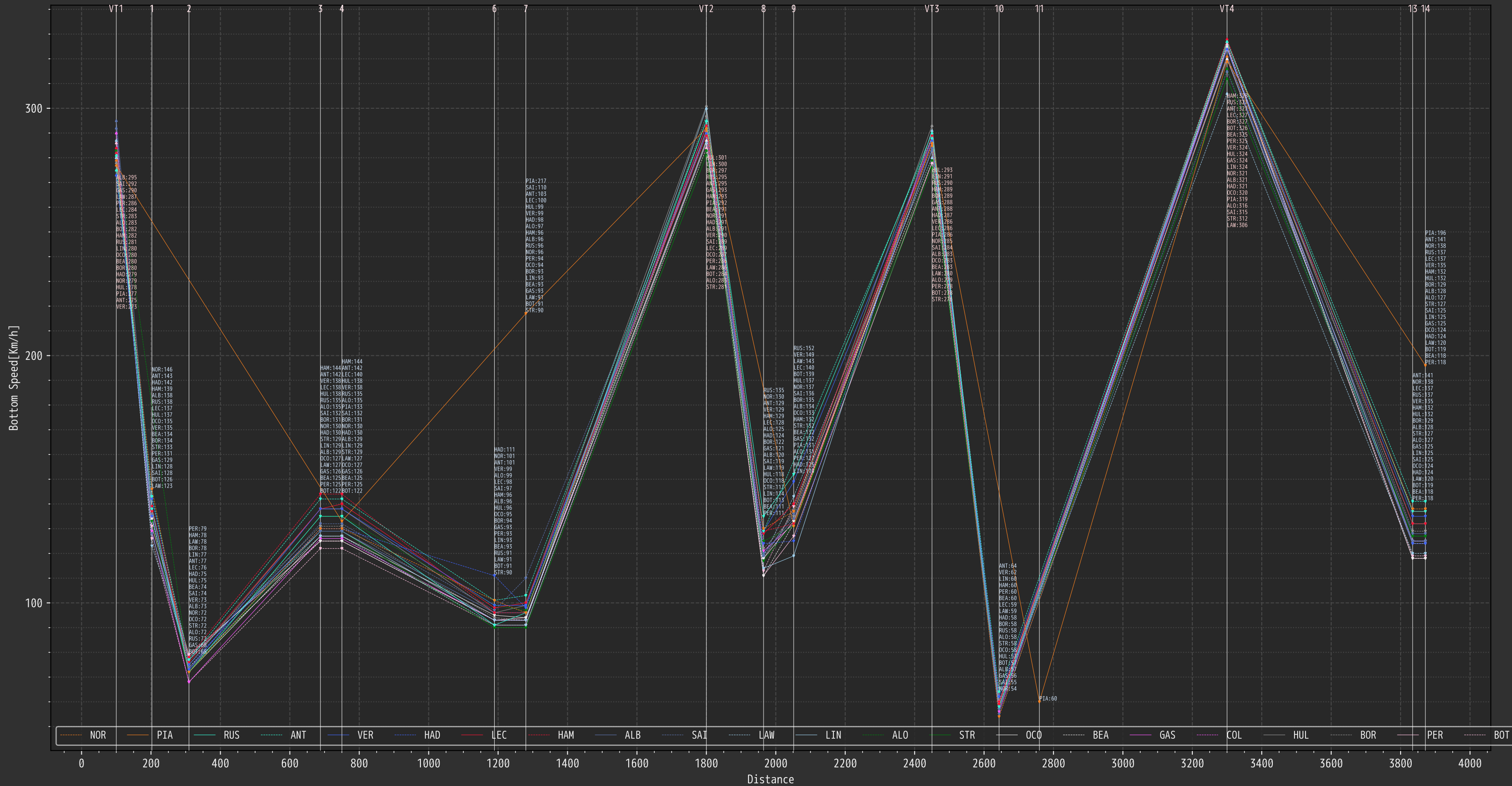
2026 Rd05 Canadian Grand Prix Practice 1 ファステストラップの各コーナーのボトムスピード(スロットル全開時を除く) + Virtual Speedtrap
