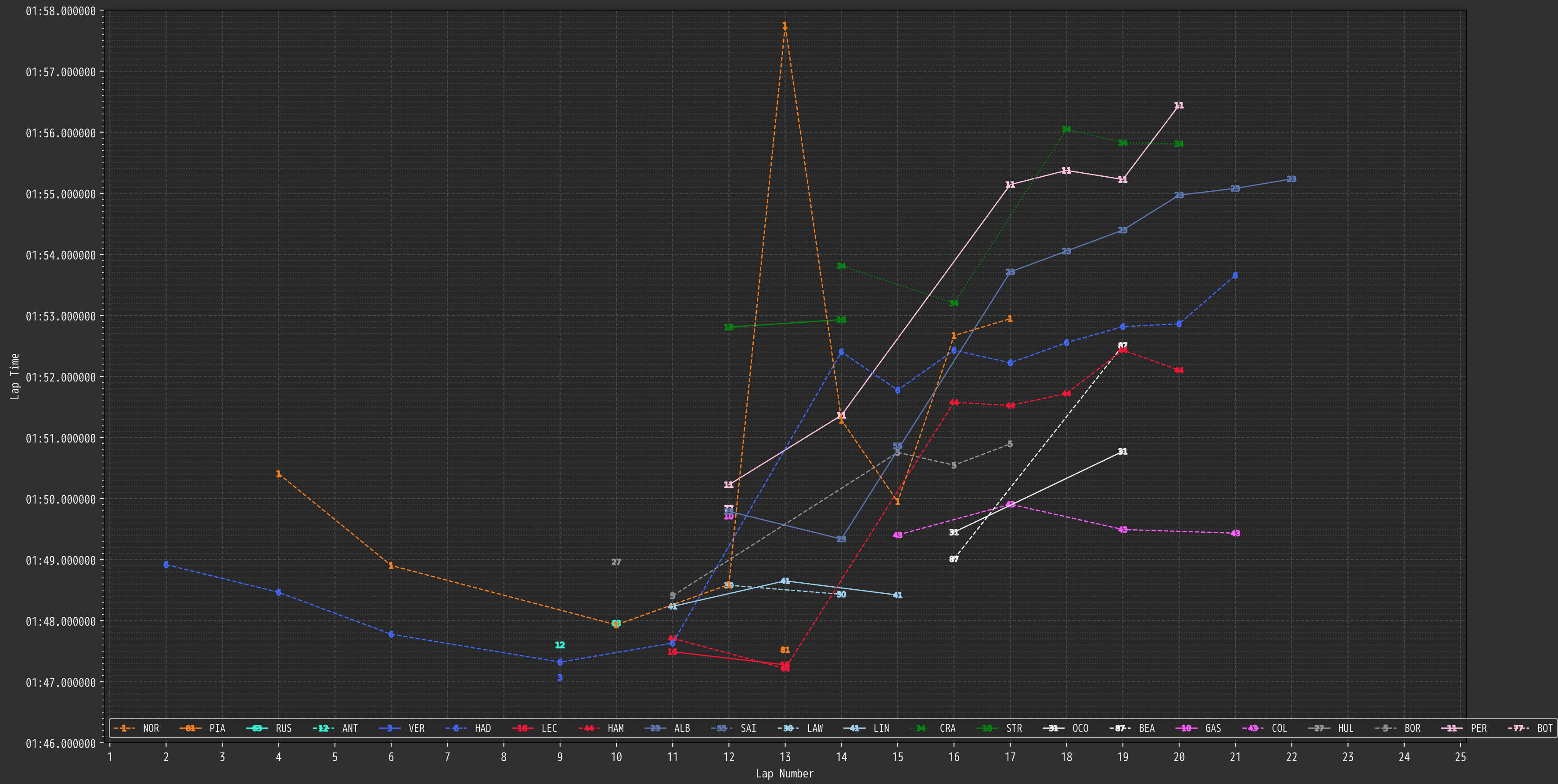
2026 Rd10 Belgian Grand Prix Practice 1 SOFTタイヤのラップタイム (1:58.000までのタイムを抽出)
