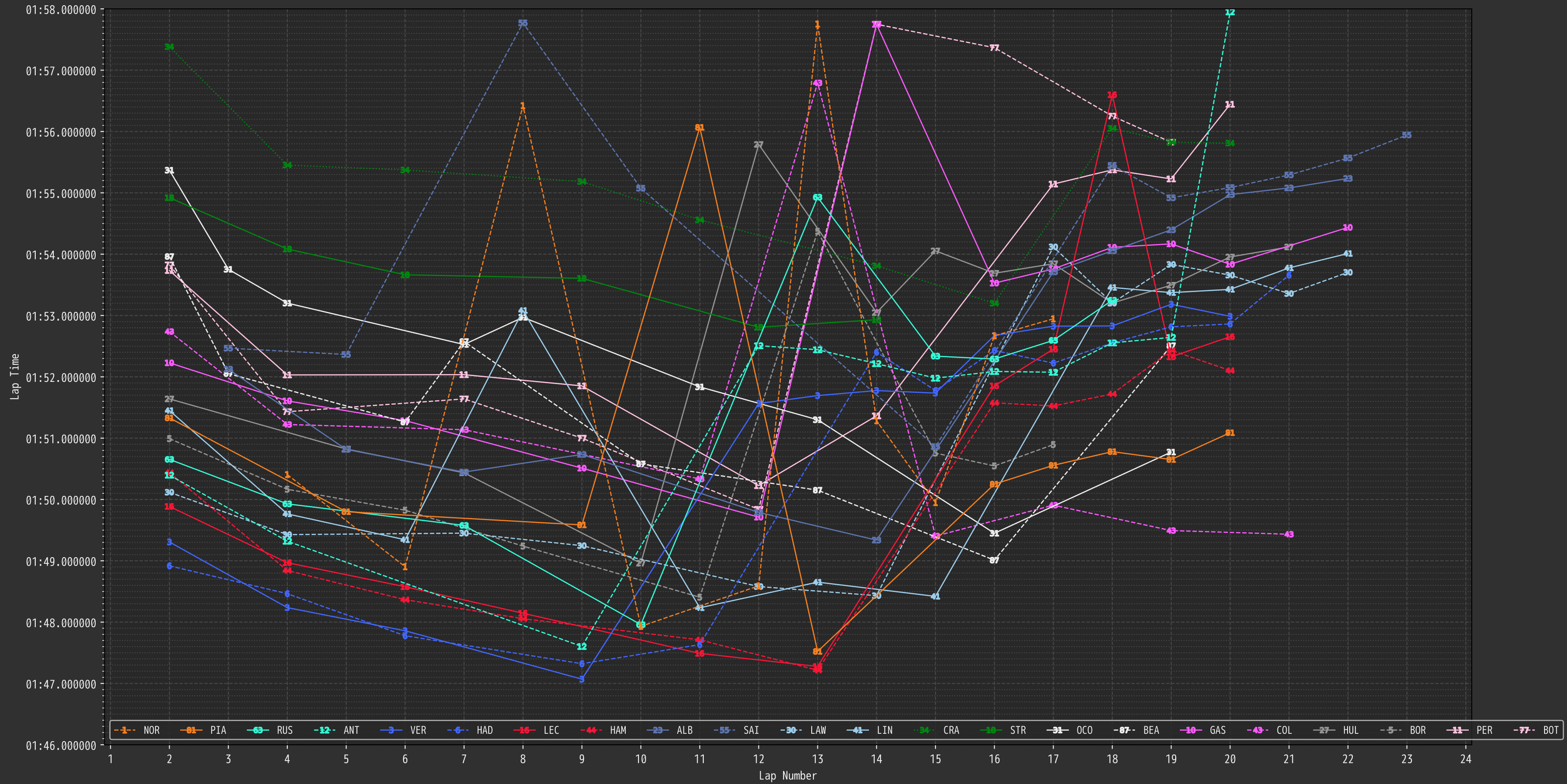
2026 Rd10 Belgian Grand Prix Practice 1 ラップタイム (1:58.000までのタイムを抽出)
