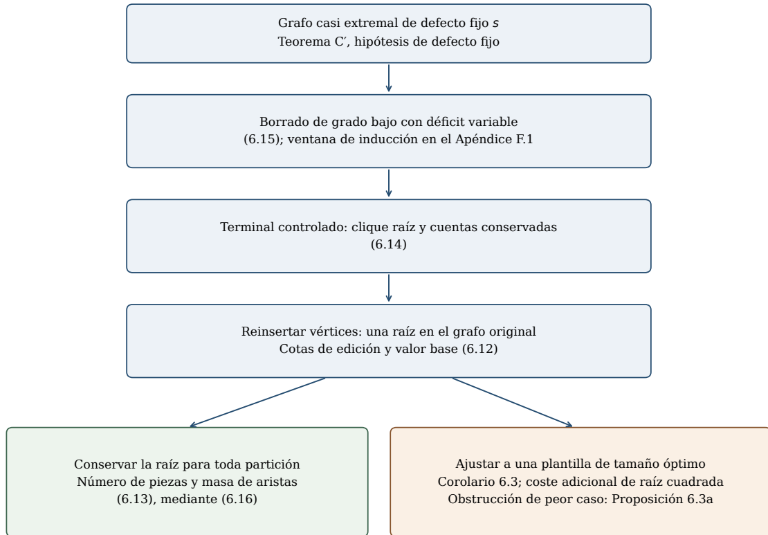
Figura 3: Estructura de la prueba de estabilidad con una misma raíz para defecto fijo. Teorema C': el borrado de vértices de grado bajo alcanza el terminal controlado, y la reinsertión transporta su raíz al grafo original. Las cuentas conservadas controlan entonces toda partición sobre esa misma raíz. Ajustar el tamaño para obtener una plantilla óptima es un paso separado (Corolario 6.3), cuyo coste de raíz cuadrada ilustra la Proposición 6.3a. El diagrama es esquemático; el Apéndice F.1 proporciona la ventana de inducción.
