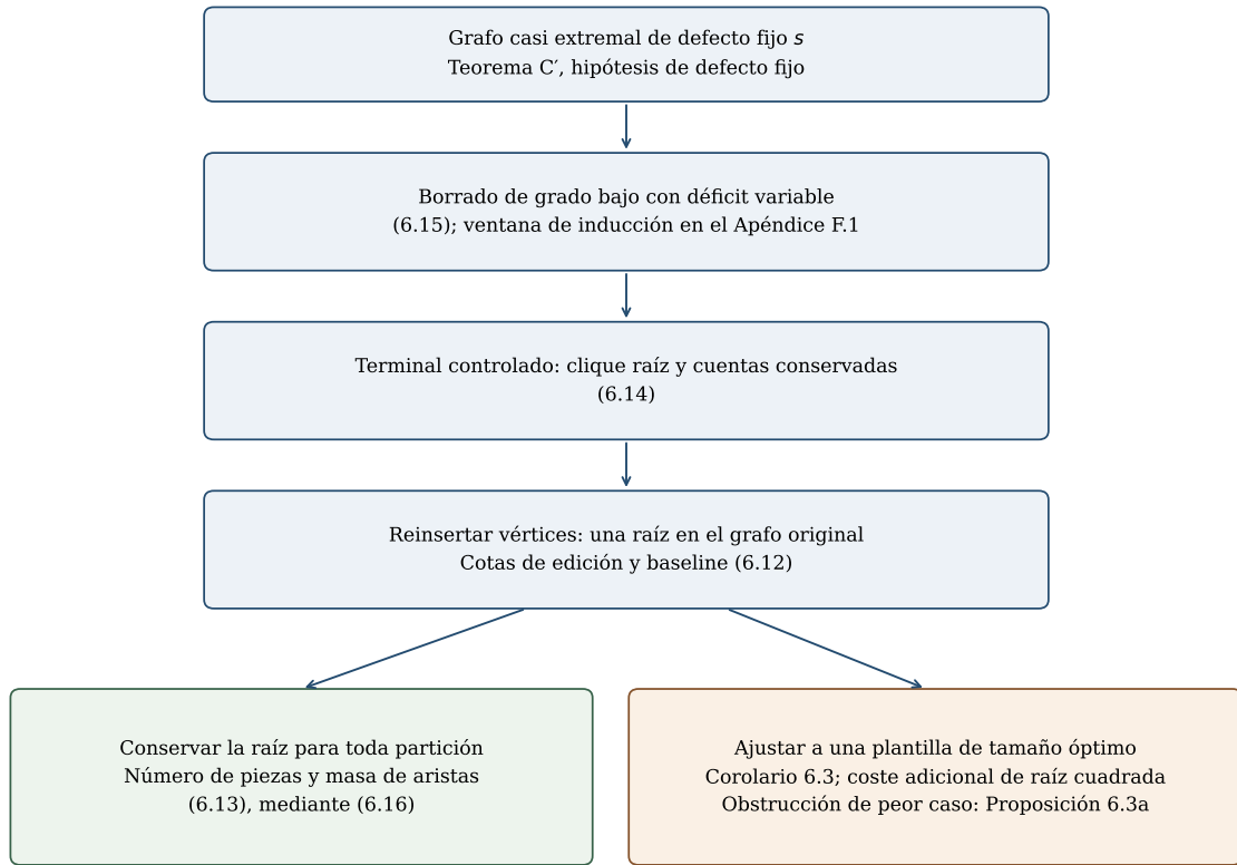
Figura 3: Estructura de la prueba de estabilidad con una misma raíz para defecto fijo. Teorema C': el borrado de vértices de grado bajo alcanza el terminal controlado, y la reinsertación transporta su raíz al grafo original. Las cuentas conservadas controlan entonces toda partición sobre esa misma raíz. Ajustar el tamaño para obtener una plantilla óptima es un paso separado (Corolario 6.3), cuyo coste de raíz cuadrada ilustra la Proposición 6.3a. El diagrama es esquemático; el Apéndice F.1 proporciona la ventana de inducción.
