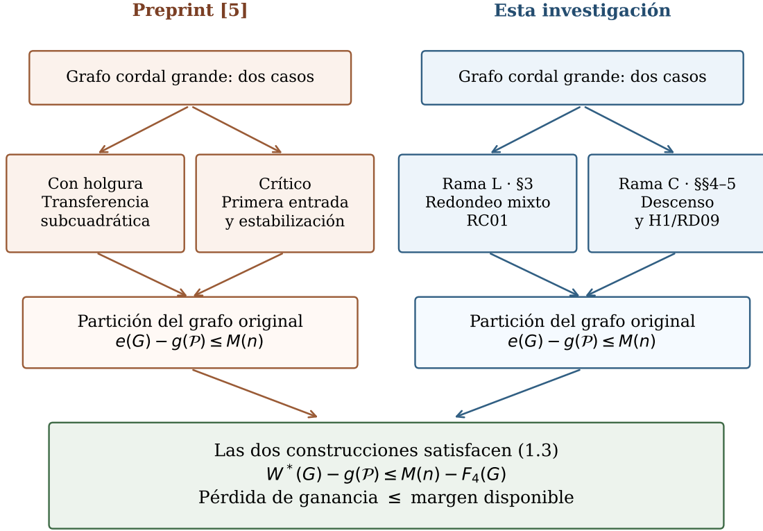
Figura 3: Comparación de mecanismos. El preprint [5] y esta investigación separan dos casos alternativos y construyen una partición que cumple (1.3). Las flechas indican implicaciones hacia la conclusión, no el paso de un régimen al otro. Los localizadores de la columna izquierda están en la Sección 8.
