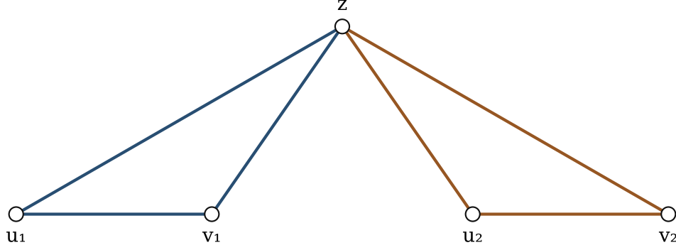
Figura 2: Dos bases disjuntas con un anfitrión común producen dos triángulos que comparten un vértice, pero ninguna arista. Esta es la unidad física utilizada en las asignaciones por clases de color.
