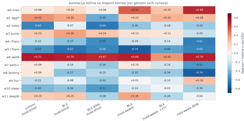
Figure 3: Korelacija vrednosti svake težine sa postignutom stopom (tet/100), preko svih arhiviranih genoma svakog runa (rani nisko-stopni genomi uključeni). Dubina bunara ( w_6 ) i kazna za prelaze po koloni ( w_5 ) su najstabilniji prediktori uspeha (neophodan bunar i „čist“ zid od gomile), dok se uloga ostalih težina razlikuje po grani razvoja.
