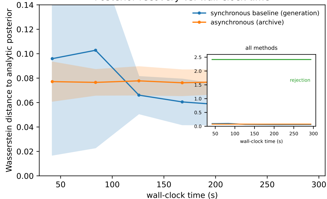
Posterior recovery vs. wall-clock time
