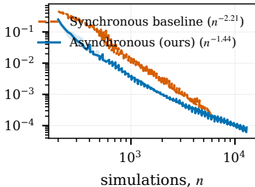
(d) Cellular Potts, 2-D, 13 s
