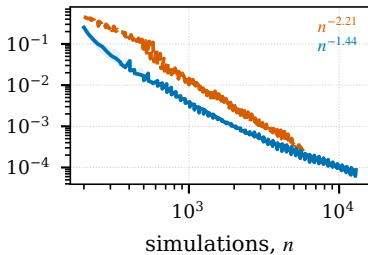
(d) Cellular Potts, 2-D, 13 s
