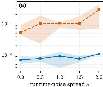
posterior-mean error
