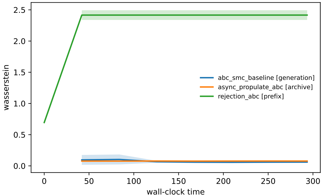
Posterior quality vs. wall-clock time
