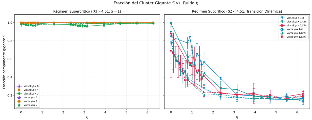
Figure 3: Fracción del cluster gigante S en función del ruido angular \eta . Panel izquierdo: régimen supercrítico ( \rho = 2, 4, 8 , N = 200, 400, 800 ), donde S \approx 1 . Panel derecho: régimen subcrítico ( \rho = 1/\pi, 1/(2\pi), 1/(3\pi) , N = 32, 16, 11 ), donde S(\eta) exhibe la desintegración dinámica del cluster con el ruido.
