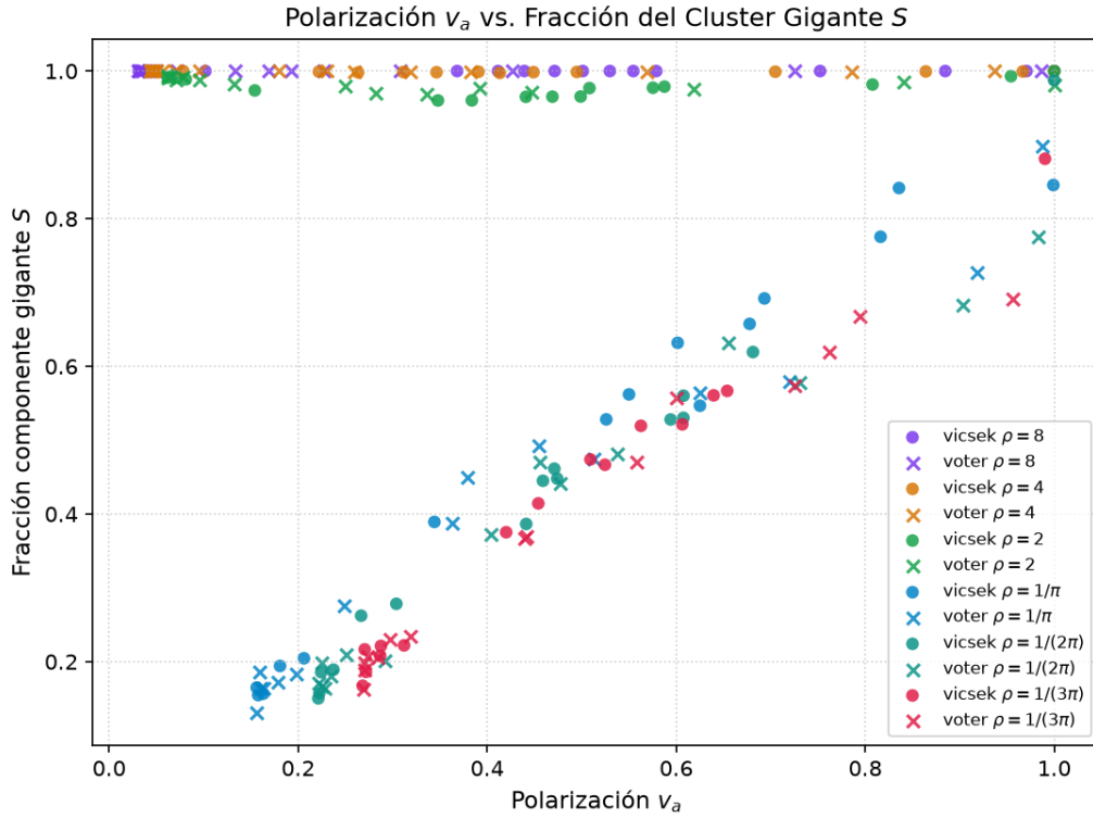
Figure 5: Polarización v_a vs. fracción del cluster gigante S , distinguiendo las densidades supercríticas ( \rho = 2, 4, 8 ) y subcríticas ( \rho = 1/\pi, 1/(2\pi), 1/(3\pi) ) para ambos modelos de interacción.
