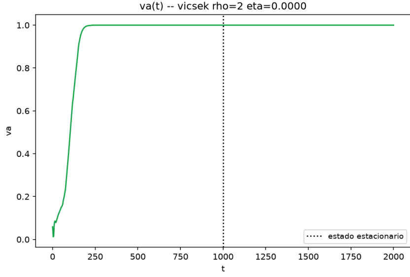
Figure 5: Evolución temporal de v_a , modelo de Vicsek, \rho = 2 , \eta = 0 . La línea vertical punteada marca el inicio de la ventana de estado estacionario (50% de los pasos descartado como transitorio).
