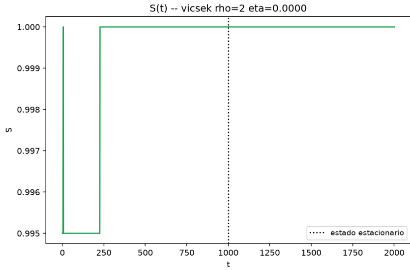
Figure 7: Evolución temporal de S , modelo de Vicsek, \rho = 2 , \eta = 0 .
