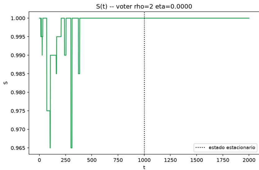
Figure 8: Evolución temporal de S , modelo de votante, \rho = 2 , \eta = 0 .
