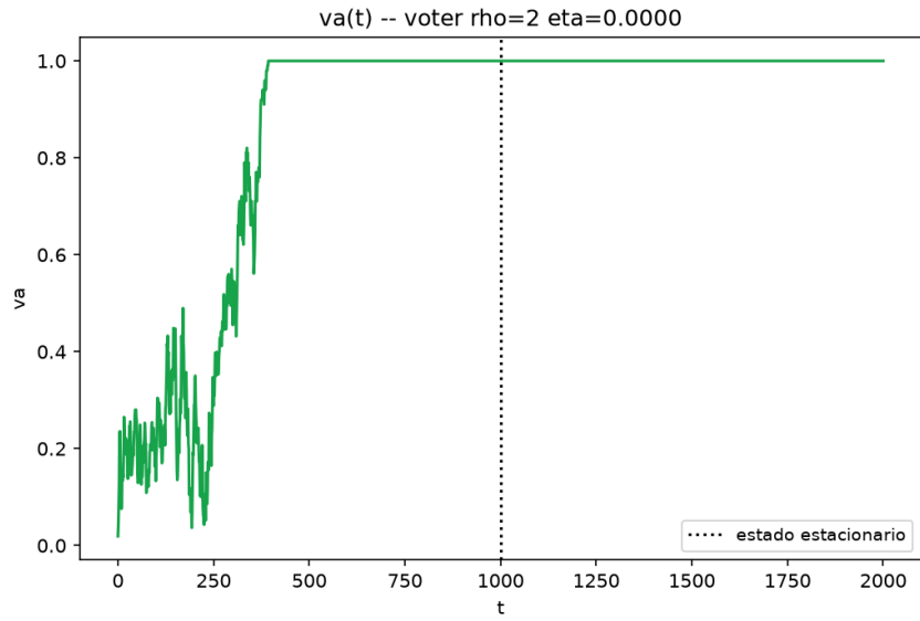
Figure 6: Evolución temporal de v_a , modelo de votante, \rho = 2 , \eta = 0 , con el mismo criterio de corte que la Fig. 5.
