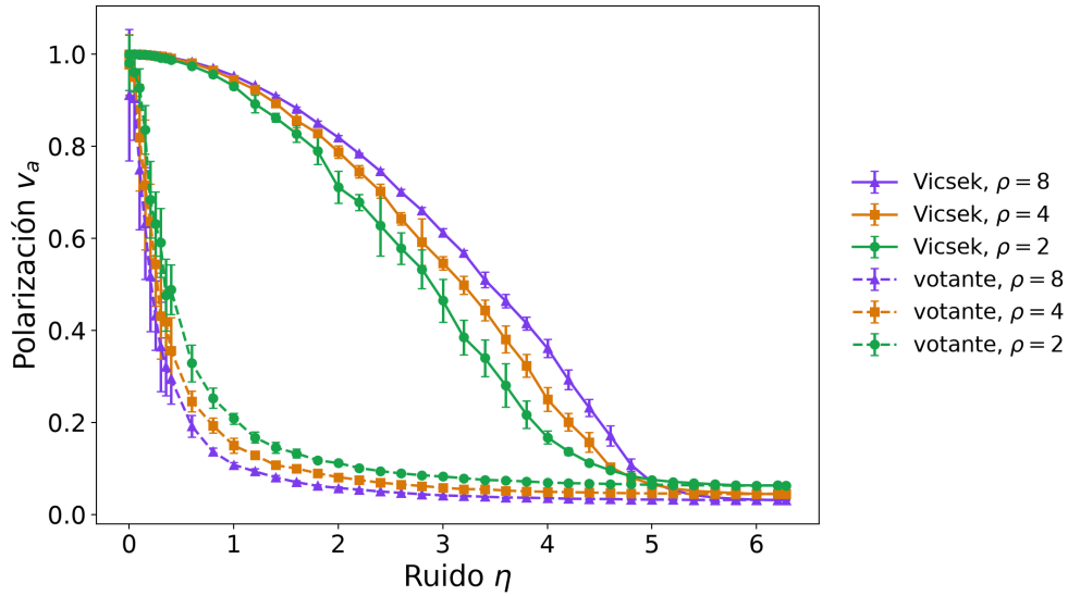
Figura 6: Polarización media de estado estacionario v_a en función de la amplitud del ruido angular \eta , para \rho \in \{2, 4, 8\} ( N = 200, 400 y 800 ) y ambos modelos de interacción (Vicsek: línea sólida; votante: línea de trazos). Parámetros comunes: L = 10 , r_c = 1 , v_0 = 0,03 , \Delta t = 1 , 2000 pasos por corrida, promedio sobre el 50 % final de cada corrida. Barras de error: desvío estándar entre K = 5 semillas independientes por punto.
