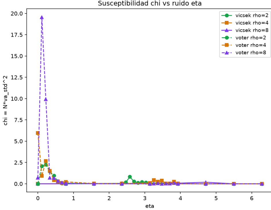
Figure 9: Susceptibilidad \chi(\eta) = N \cdot \text{Var}(v_a) en función del ruido angular \eta .
