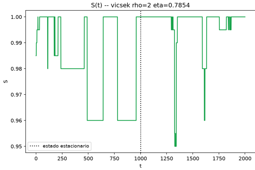
Figure 7: Evolución temporal de S , modelo de Vicsek, \rho = 2 , \eta = 0.7854 .
