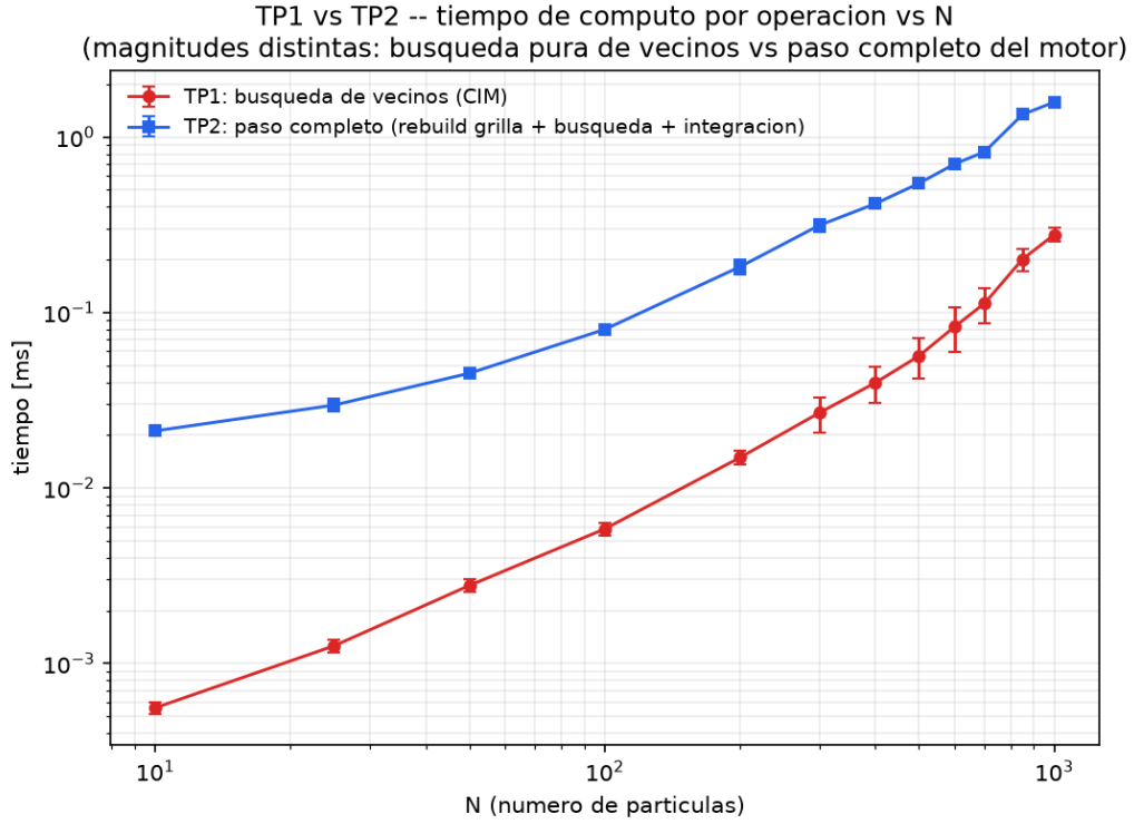
Figure 10: Tiempo de cómputo por operación vs. número de partículas N (escala log-log): búsqueda de vecinos del CIM (TP1, L = 20 ) vs. paso completo del motor incl. escritura de trayectoria (TP2, L = 10 ). Magnitudes y densidades distintas, no directamente comparables en valor absoluto.
