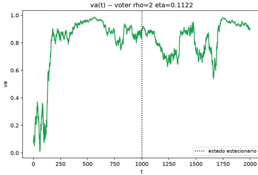
Figure 6: Evolución temporal de v_a , modelo de votante, \rho = 2 , \eta = 0.1122 , con el mismo criterio de corte que la Fig. 5.
