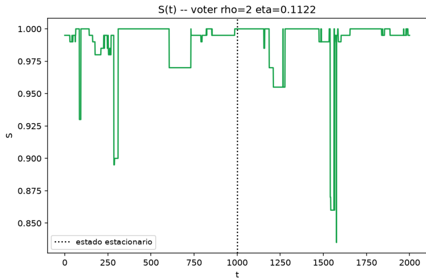
Figure 8: Evolución temporal de S , modelo de votante, \rho = 2 , \eta = 0.1122 .
