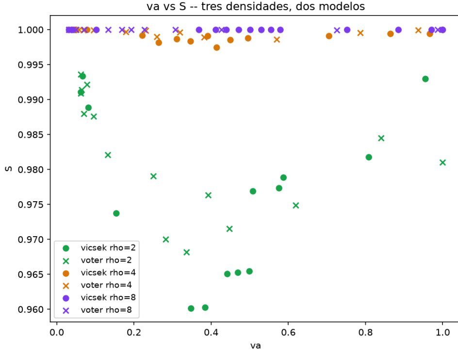
Figure 4: Polarización v_a vs. fracción del cluster gigante S , distinguiendo las tres densidades y ambos modelos.
