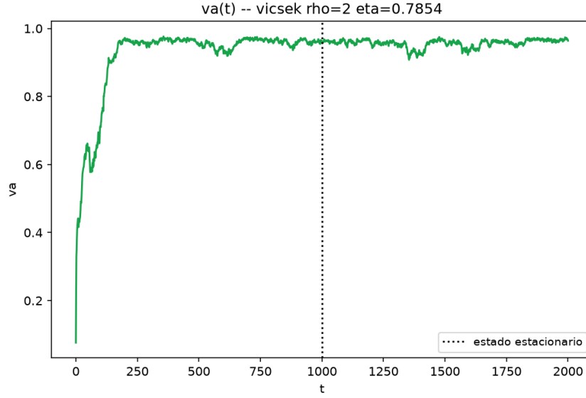
Figure 5: Evolución temporal de v_a , modelo de Vicsek, \rho = 2 , \eta = 0.7854 . La línea vertical punteada marca el inicio de la ventana de estado estacionario (50% de los pasos descartado como transitorio).
