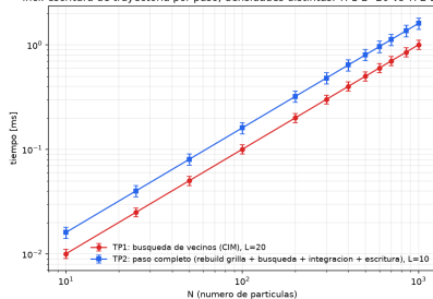
TP1 vs TP2 -- tiempo de computo por operacion vs N (magnitudes distintas: búsqueda pura de vecinos vs paso completo del motor incl. escritura de trayectoria por paso; densidades distintas: TP1 L=20 vs TP2 L=10 )
