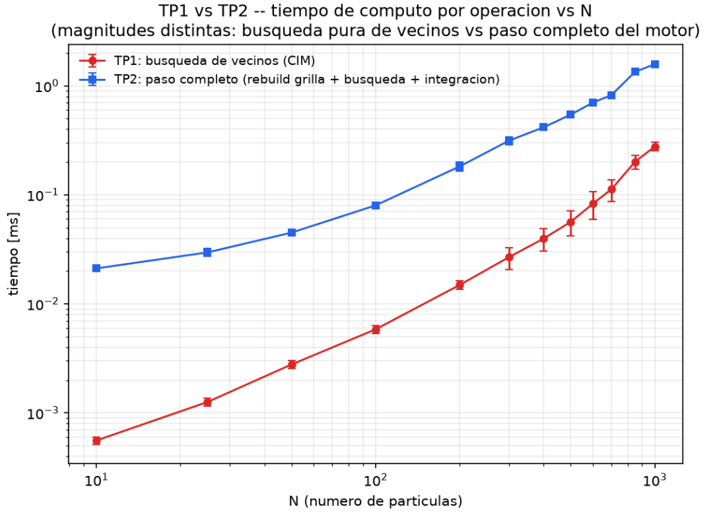
Figure 9: Tiempo de cómputo por operación vs. número de partículas N (escala log-log): búsqueda de vecinos del CIM (TP1) vs. paso completo del motor (TP2). Magnitudes distintas, no directamente comparables en valor absoluto.
