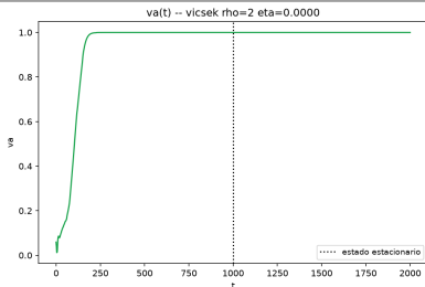
Vicsek v_a(t)
