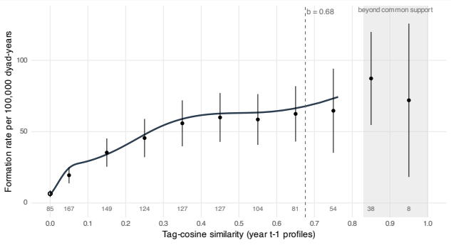
Curva: predicciones medias del logit con spline. Puntos: tasas ajustadas del logit con similitud por tramos (intervalos de confianza diádicos).
