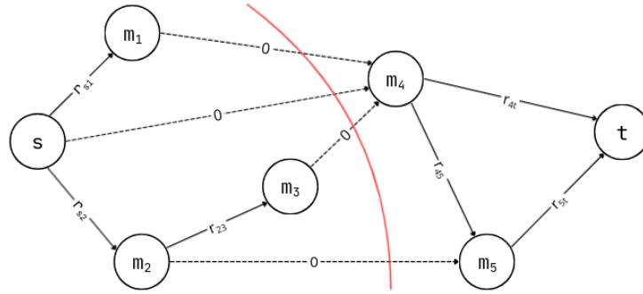
Figura 2: Corte mínimo de la red de relaciones
