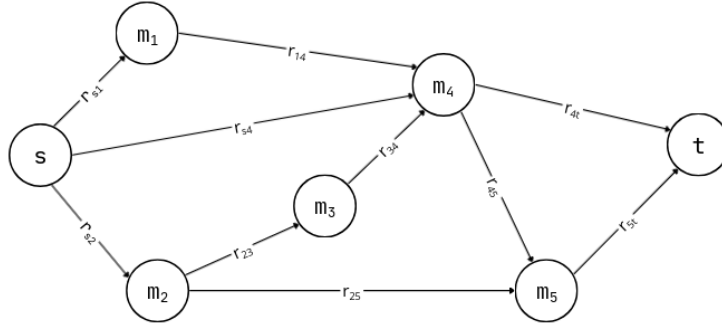
Figura 1: Ejemplo de red de flujo de relaciones
